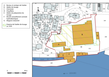
Plan-masse et de situation. Extrait du plan cadastral, 2015, section AN. Dess. Mathias Papigny IVR43_20152502650NUDA
