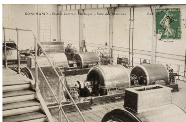
Ronchamp - Station Centrale électrique - Salle des machines. Phot. Jérôme Mongreville IVR43_20057000618NUCA
