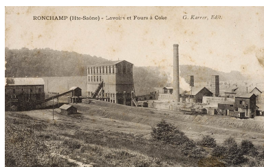
Ronchamp (Hte-Saône). - Lavoires et fours à coke. Phot. Jérôme Mongreville IVR43_20057000641NUCA
