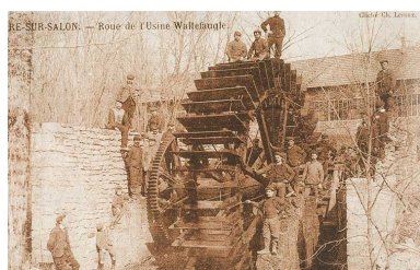
Dampierre sur Salon. - Roue de l'usine Waltefaugle. Phot. Jérôme Mongreville, Autr. Ch. (photographe) Leroux IVR43_20097000077NUC2A
