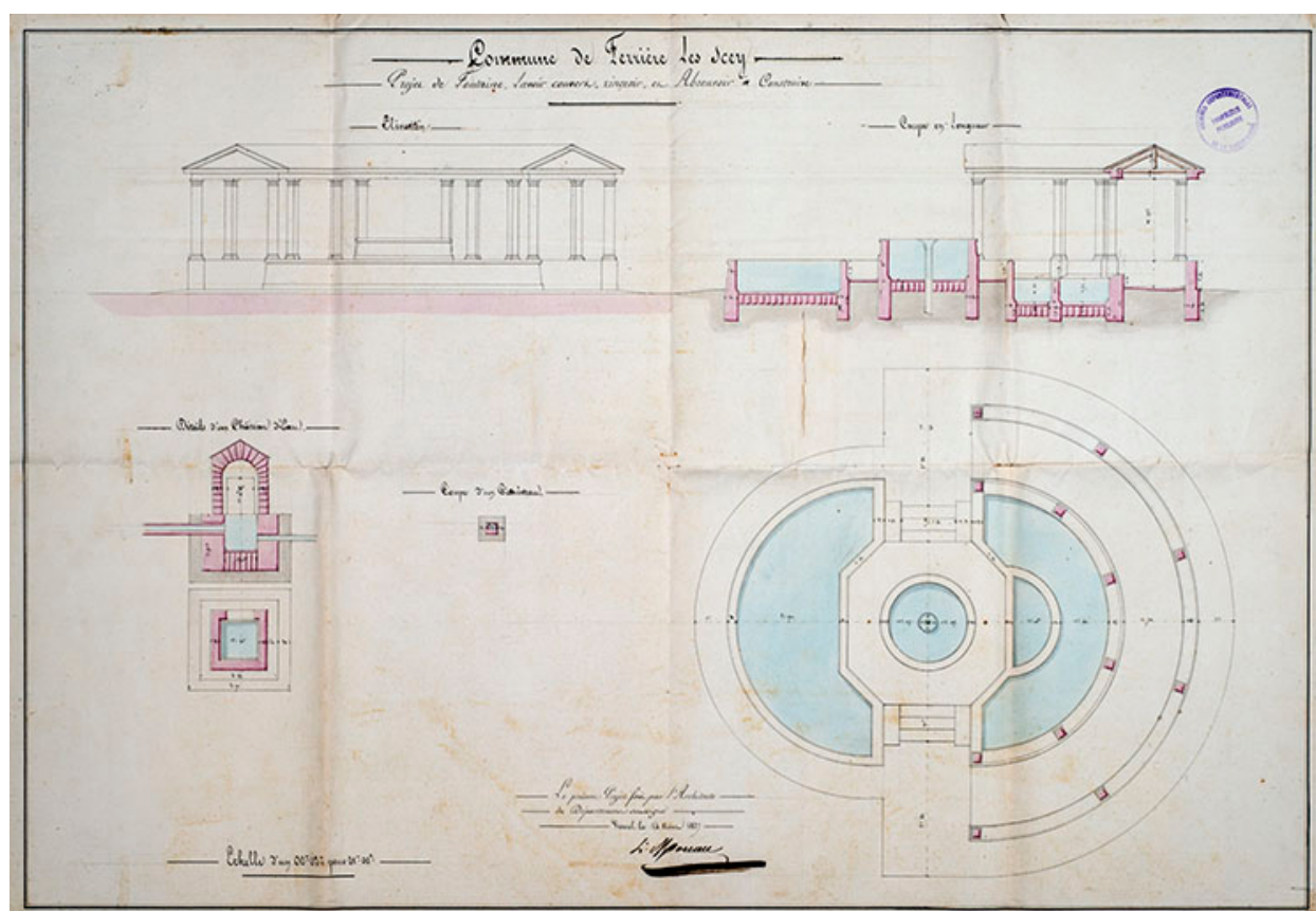
Projet de fontaine, lavoir couvert, ringoir et abreuvoir à construire : plan, coupe élévation (1827).
