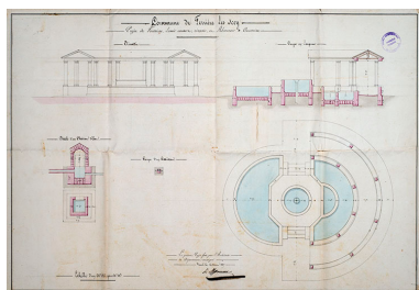
Projet de fontaine, lavoir couvert, rîncioir et abreuvoir à construire : plan, coupe élévation (1827).
