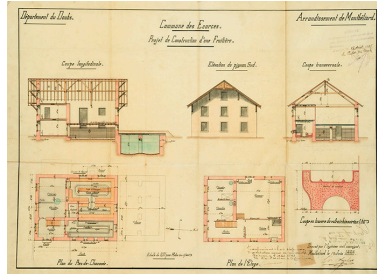
Commune des Écorces. Projet de construction d'une fruitière, 1898. Phot. Jérôme Mongreville, Autr. Charles-Frédéric Surleau IVR43_20152500567NUC4A
