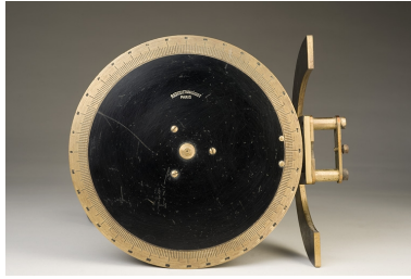
Le disque horizontal, avec son limbe et le nom du fabricant. Phot. Marc Loukachine IVR43_20122500060NUC4A
