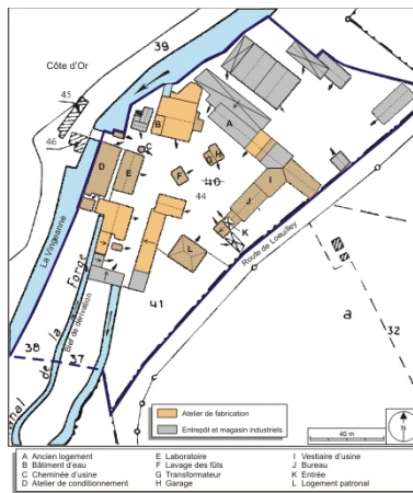
Plan-masse et de situation. Extrait du plan cadastral numérisé, 2008, section ZE, 1:2000 agrandi à 1:1250. Source : Direction générale des Finances Publiques - Cadastre ; mise à jour : 2008.
