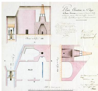
Plan, élévation et coupe du haut fourneau que se propose de
