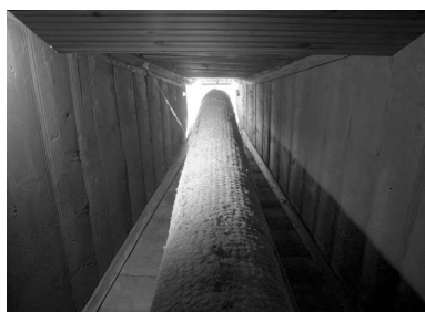
Intérieur du conduit de la cheminée en bois, un nouveau conduit isolé a été ajouté pour la cheminée actuelle.
