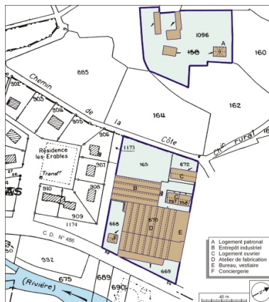
Plan-masse et de situation. Extrait du plan cadastral numérisé, 2005, section H, 1:2000 agrandi à 1:1500. Dess. André Céréza IVR43_20067000056NUDA
