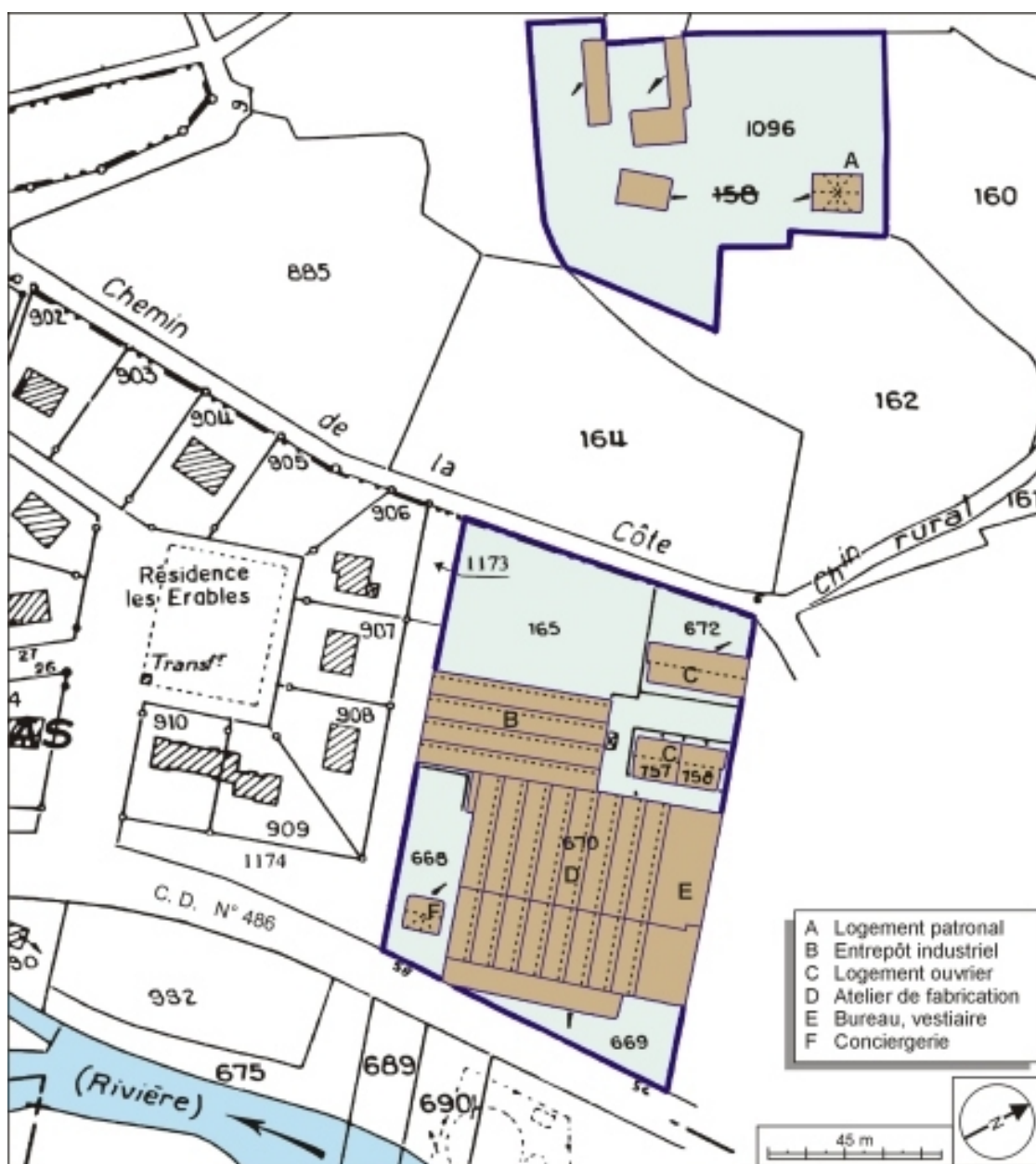
Plan-masse et de situation. Extrait du plan cadastral numérisé, 2005, section H, 1:2000 agrandi à 1:1500.
