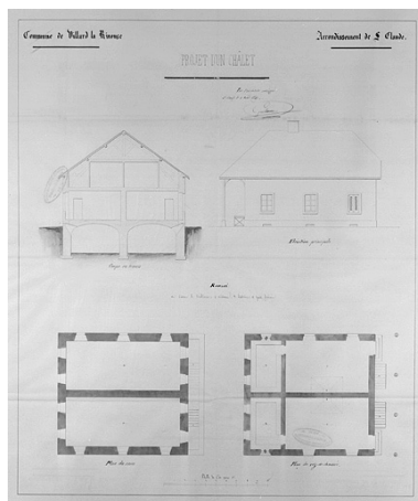
Projet d'un chalet : plan du rez-de-chaussée et des caves, façades, coupes. Phot. Jérôme Mongreville, Phot. Ernest Guillaume IVR43_19973901018V
