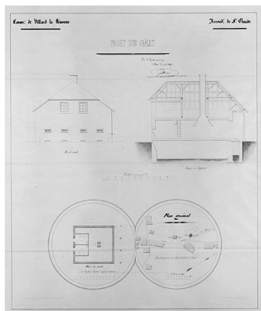
Projet d'un chalet : plan de situation, façade, coupe et plan des combles.
