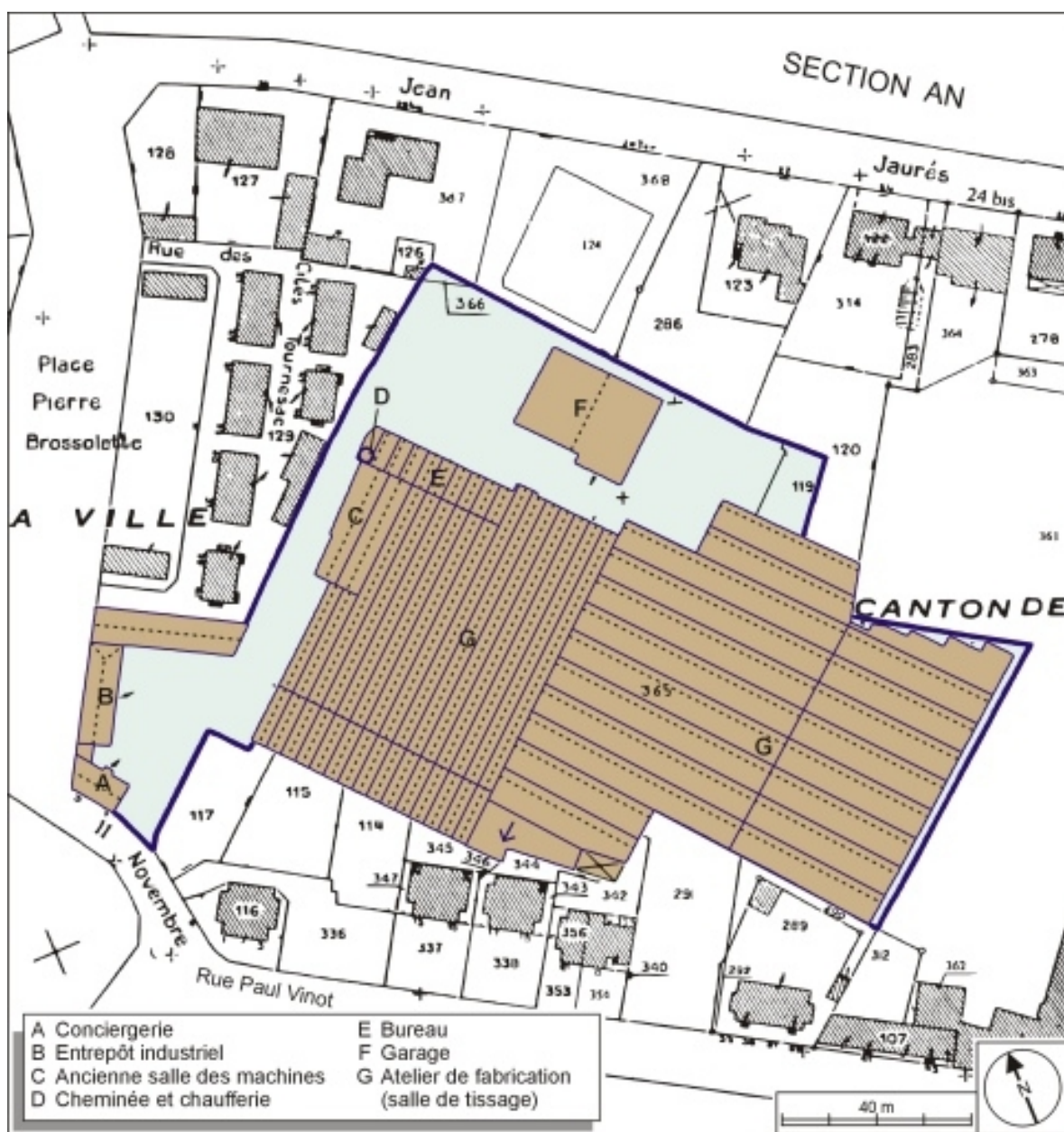
Plan-masse de l'usine. Extrait du plan cadastral numérisé, 2005, section AO, 1:1000 réduit à 1:1250.
