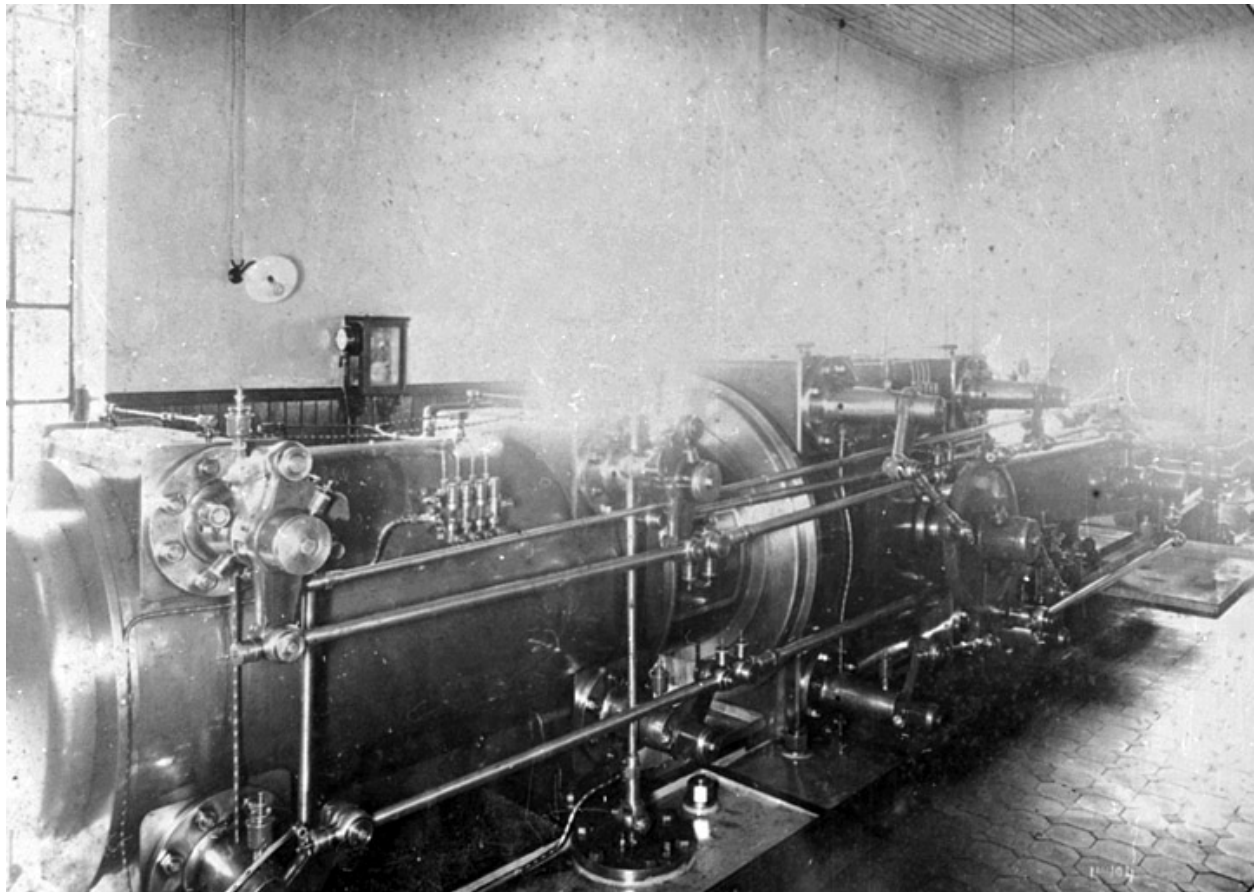
Société Anonyme de Filature et Tissage de Giromagny. Usine de la Fonderie : machine à vapeur.
