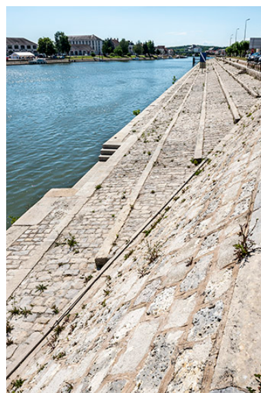
Détail de la maçonnerie du quai. Phot. Jérôme Mongreville IVR43_20197000330NUC4A
