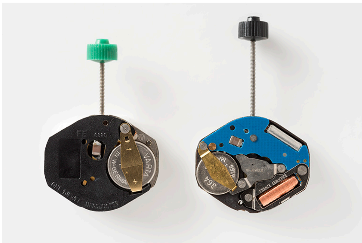
Mouvements France Ebauches FE 6320 (à gauche) et FE 6920 (à droite) : face côté fond.
