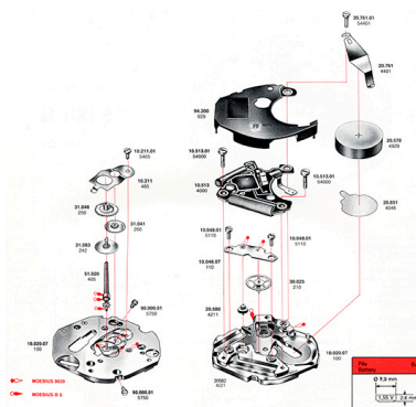
[Vue éclatée du mouvement FE 6320], 1989. IVR43_20172500284NUC4A
