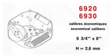
[Dessin des mouvements FE 6920 et 6930], 1989. IVR43_20172500285NUC4A
