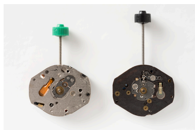
Mouvements France Ebauches FE 6320 (à gauche) et FE 6920 (à droite) : face côté cadran. Phot. Sonia Dourlot IVR43_20172500202NUC4A
