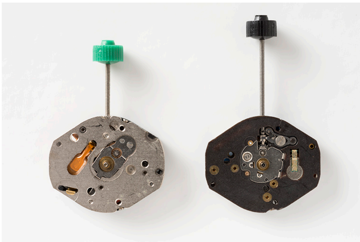
Mouvements France Ebauches FE 6320 (à gauche) et FE 6920 (à droite) : face côté cadran.
