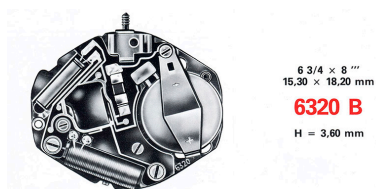
[Dessin du mouvement FE 6320 B], 1989. IVR43_20172500283NUC4A
