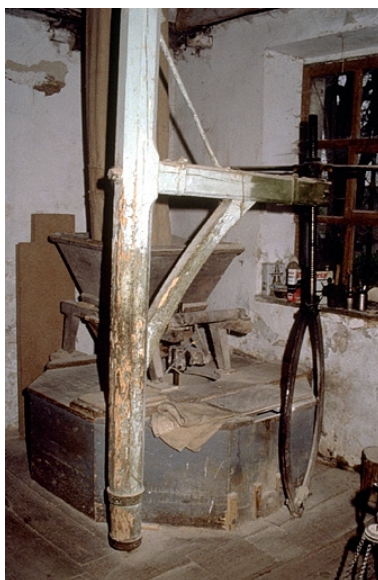
Intérieur : rez-de-chaussée, salle des meules, meules et potence.
