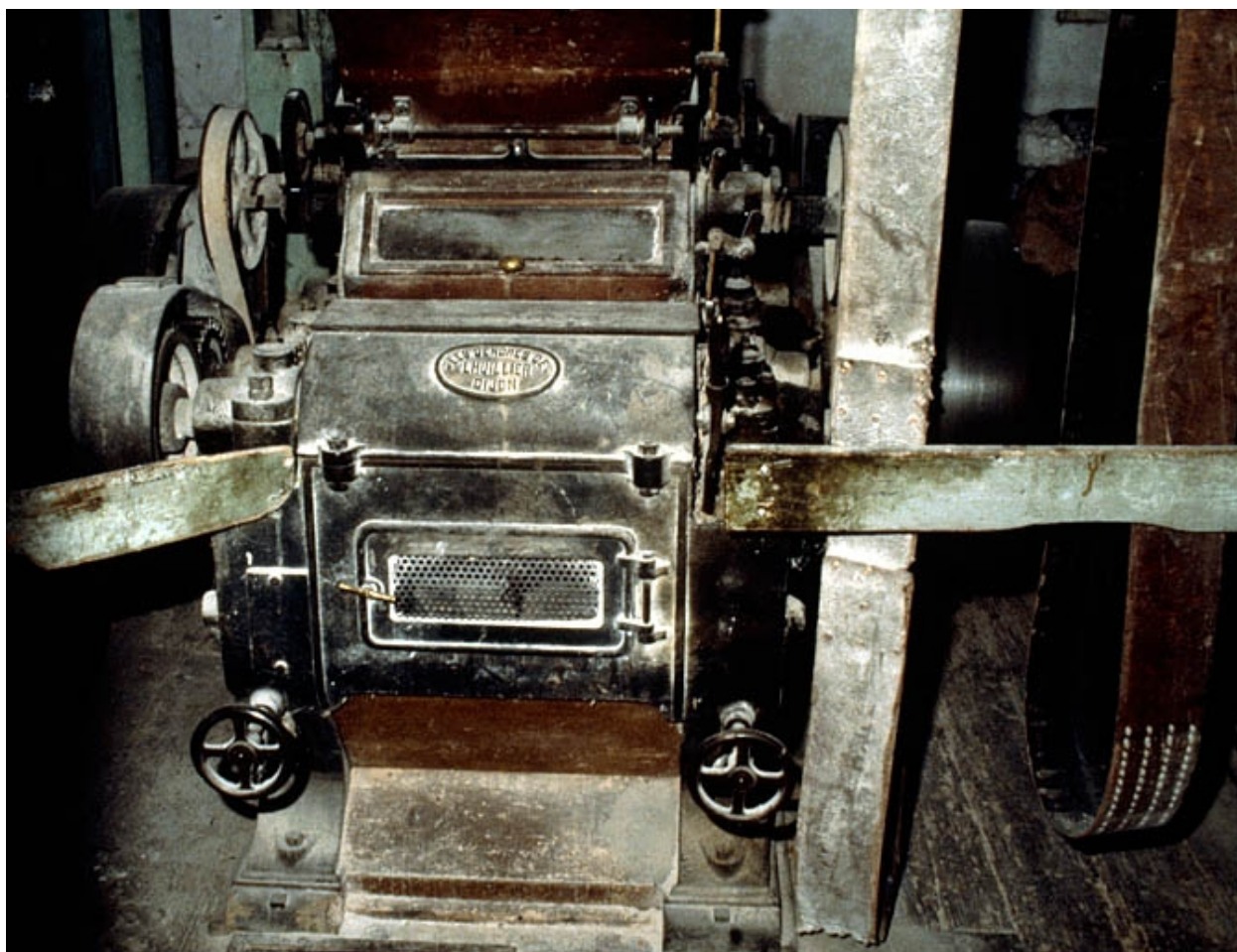
Intérieur : rez-de-chaussée, salle des meules, convertisseur vu de face.
