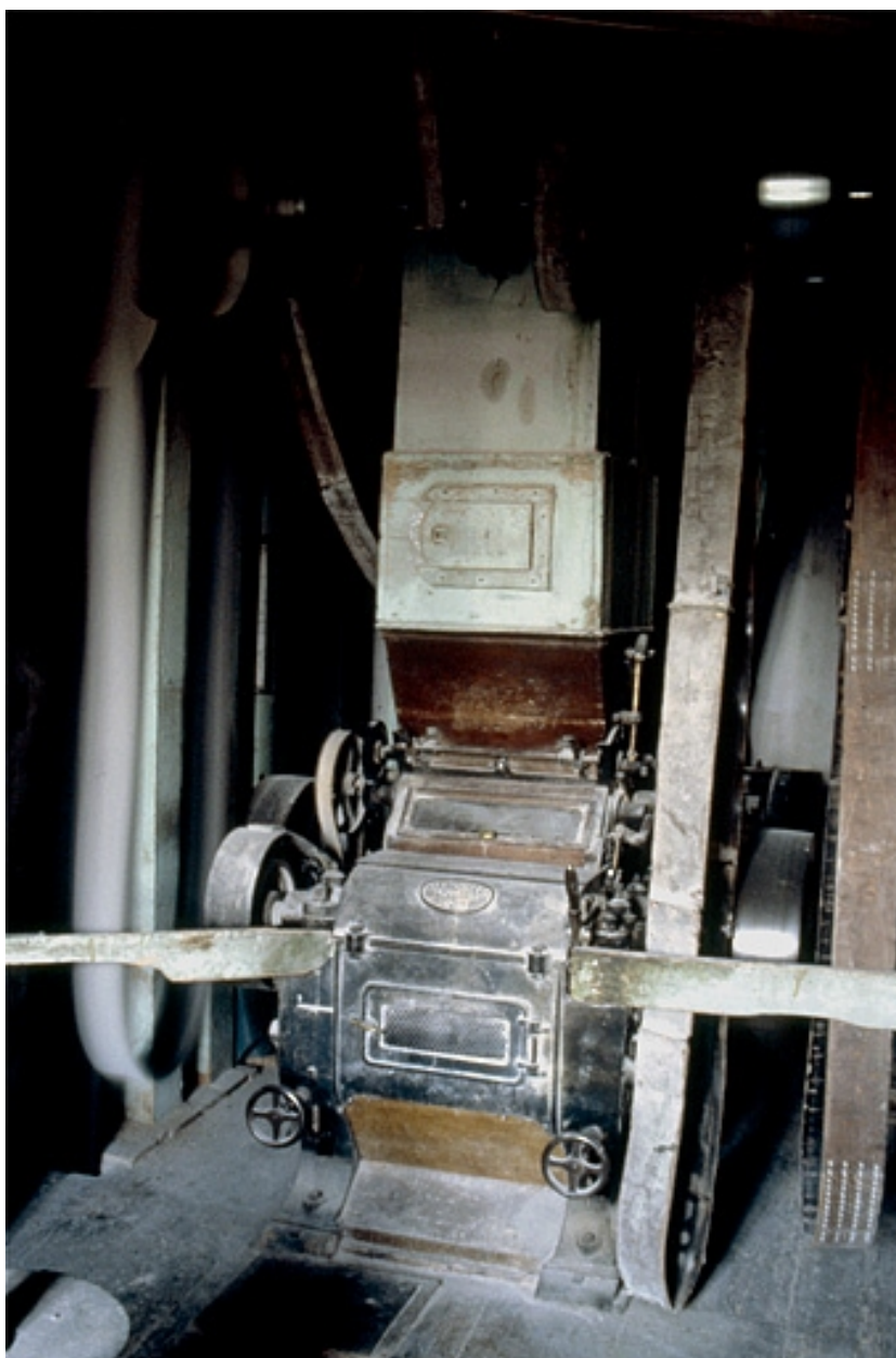
Intérieur : rez-de-chaussée, salle des meules, convertisseur vu de trois quarts.
