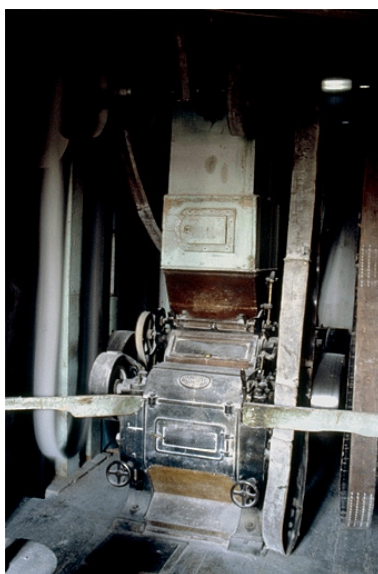
Intérieur : rez-de-chaussée, salle des meules, convertisseur vu de trois quarts. Phot. Laurent Poupard IVR43_19883900007ZA
