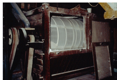
Intérieur : étage, salle de la bluterie, bluterie centrifuge. Phot. Laurent Poupard IVR43_19883900012ZA
