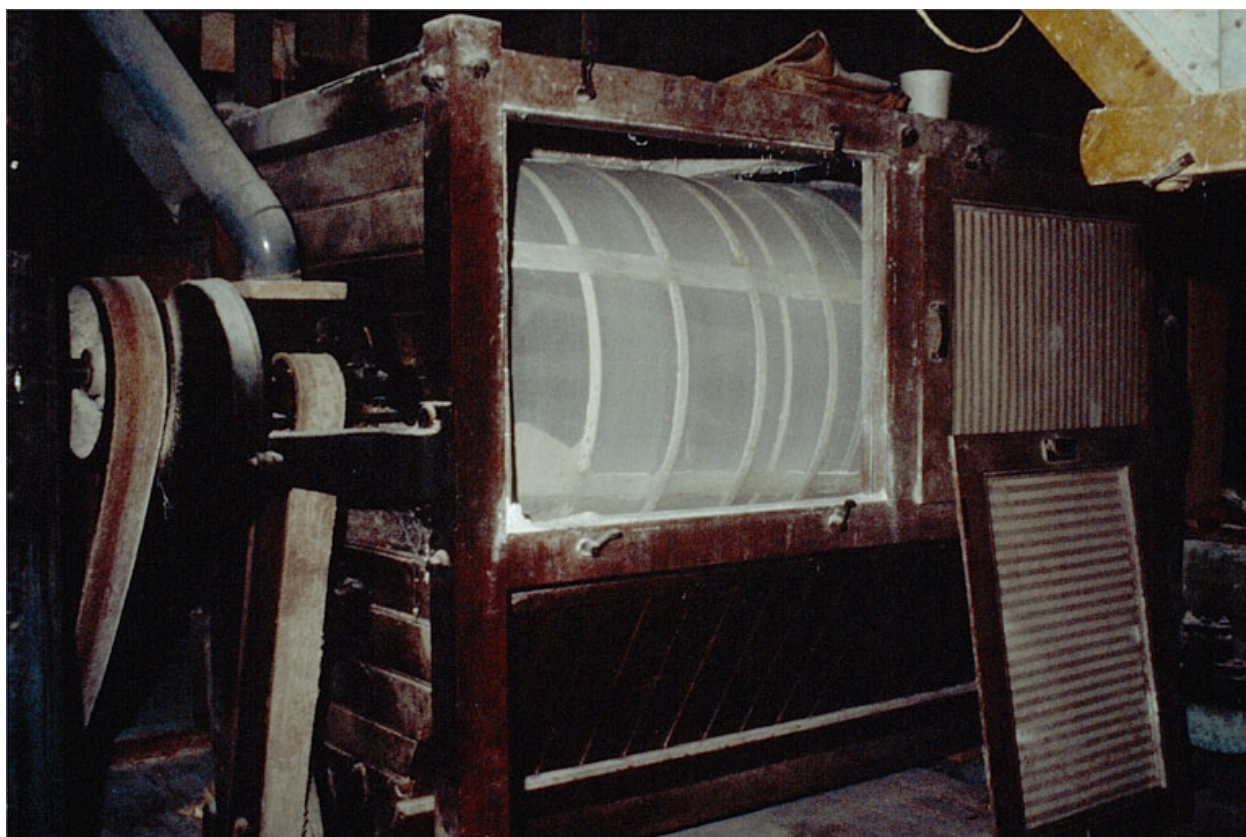
Intérieur : étage, salle de la bluterie, bluterie centrifuge.
