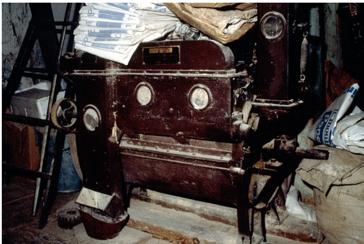
Intérieur : rez-de-chaussée, salle des meules, décortiqueuse dite floconneuse.
