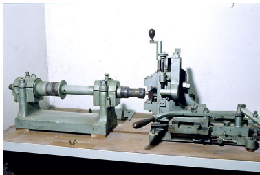
Machine à façonner (défonceuse). Phot. Jérôme Mongreville IVR43_20003901120ZA
