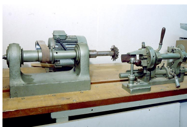
Machine à fraiser dite machine à arrondir. Phot. Jérôme Mongreville IVR43_20003901131ZA
