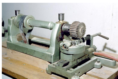
Machine à fraiser dite machine à cintrer. Phot. Jérôme Mongreville IVR43_20003901135ZA
