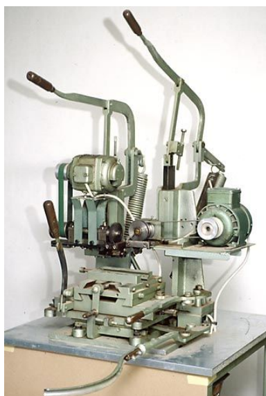
Machine à fraiser : machine à équarrir dite machine infernale. Phot. Jérôme Mongreville IVR43_20013900277ZA
