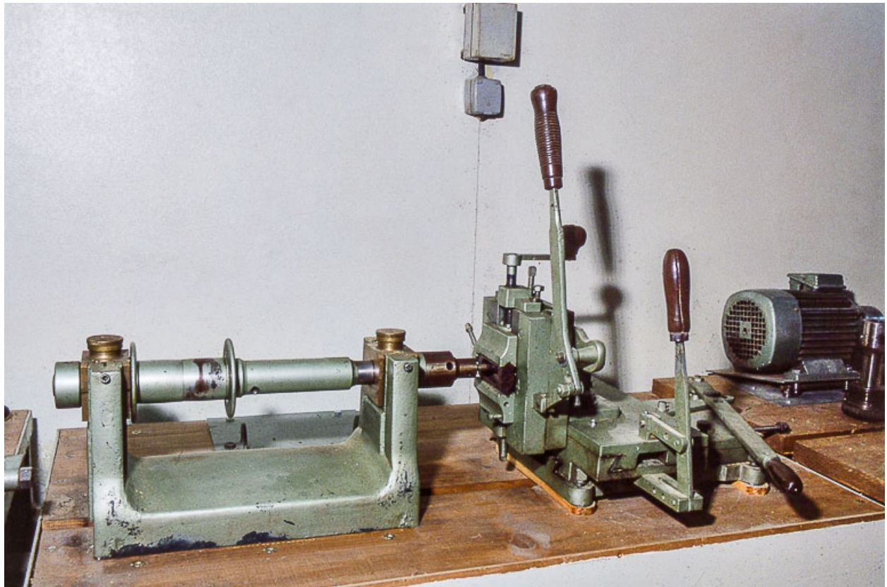
Machine à fraiser dite machine à renfoncer.
