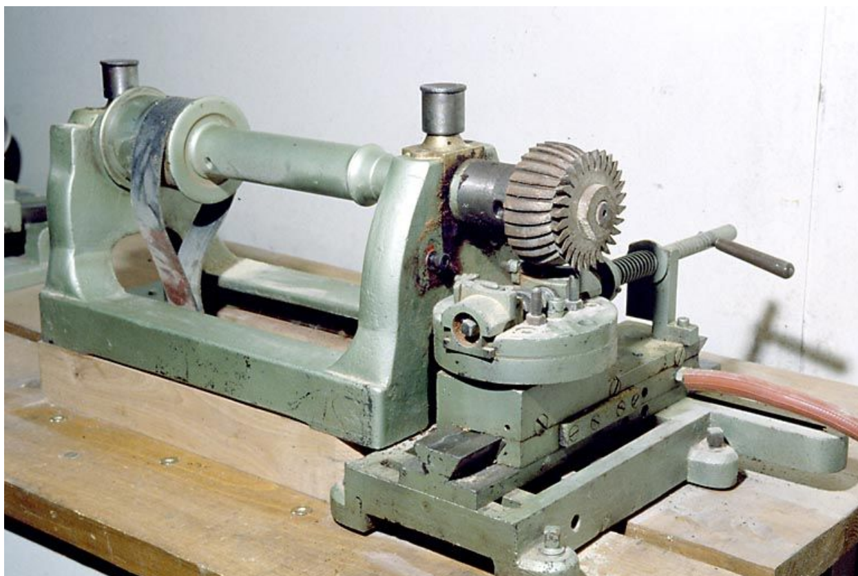
Machine à fraiser dite machine à cintrer.
