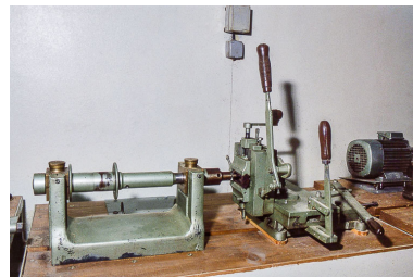
Machine à fraiser dite machine à renfoncer. Phot. Jérôme Mongreville IVR43_20003901147ZA
