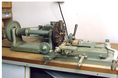
Machine à fraiser dite machine à ovaliser ou varlope. Phot. Jérôme Mongreville IVR43_20003901128ZA
