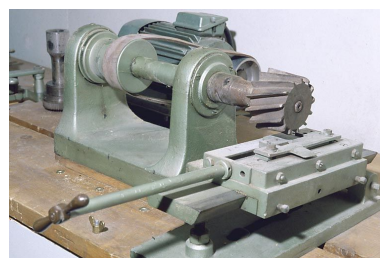
Machine à fraiser dite machine à bomber. Phot. Jérôme Mongreville IVR43_20003901133ZA
