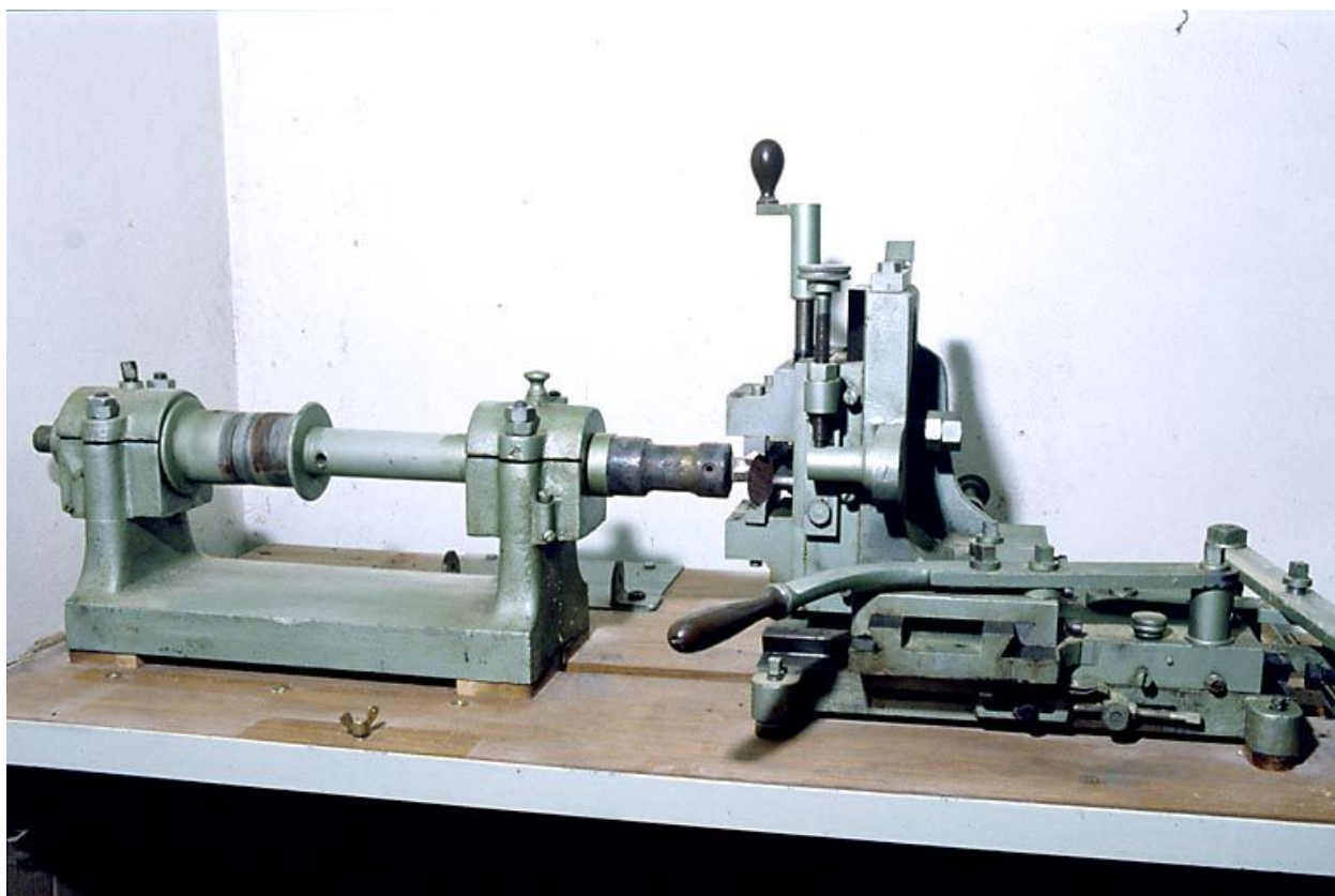
Machine à façonner (défonceuse).
