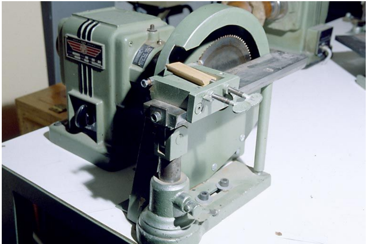
Machine à découper par scie (scie circulaire).
