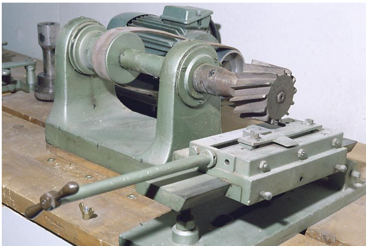
Machine à fraiser dite machine à bomber.
