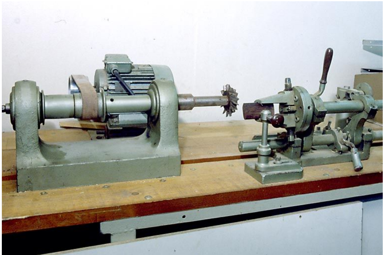
Machine à fraiser dite machine à arrondir.
