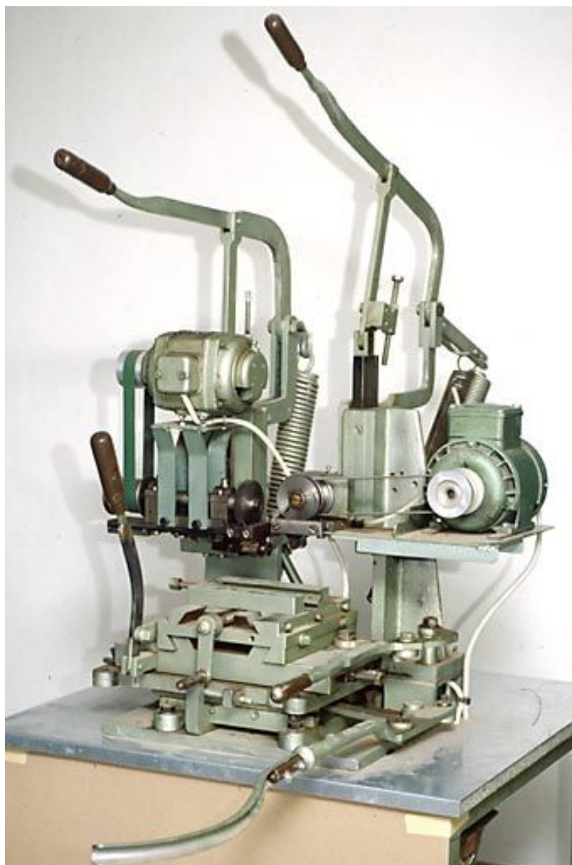
Machine à fraiser : machine à équarrir dite machine infernale.
