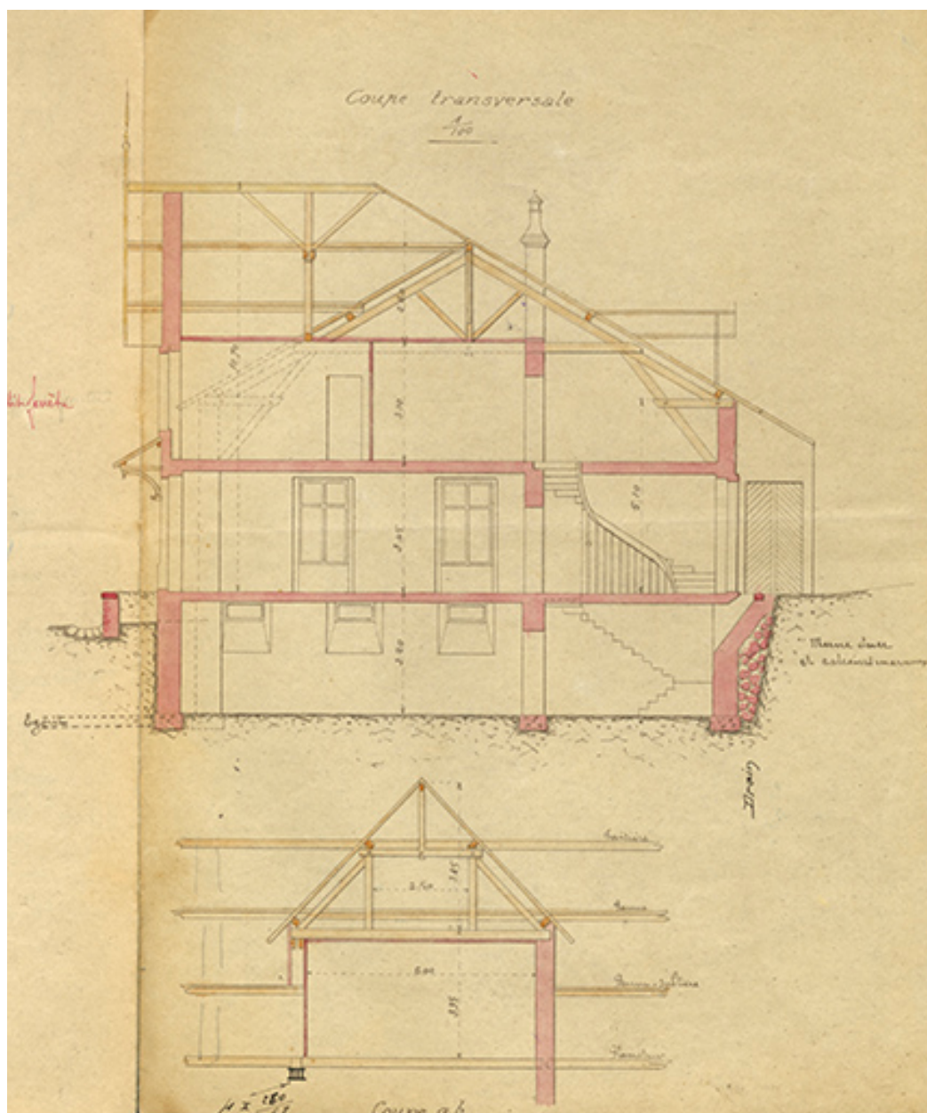
Projet de construction d'un chalet-modèle, coupe transversale, 1906.
