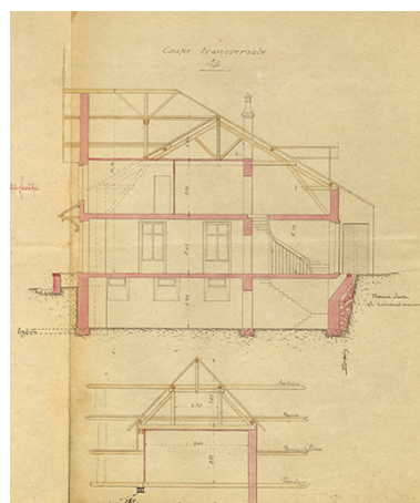
Projet de construction d'un chalet-modèle, coupe transversale, 1906. IVR43_20192500094NUC4A
