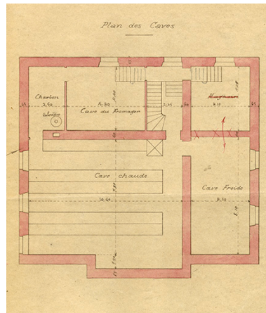
Projet de construction d'un chalet-modèle. Plan des caves, 1906. IVR43_20192500096NUC4A
