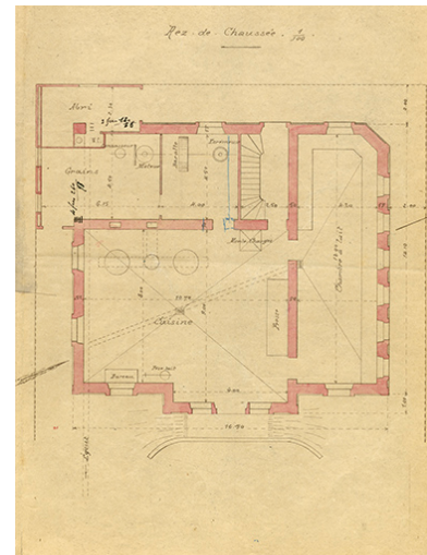
Projet de construction d'un chalet-modèle. Plan du rez-de-chaussée, 1906. IVR43_20192500097NUC4A
