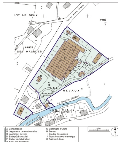
Plan-masse et de situation. Extrait du plan cadastral numérisé, 2005, section AC, 1:1000 réduit à 1:1500. Dess. André Céréza IVR43_20067000011NUDA
