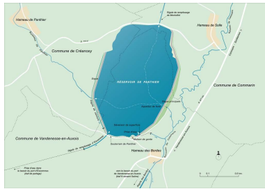
Plan schématique du réservoir. Dess. Alain Morelière IVR26_20132100089NUDA
