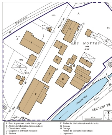
Plan-masse et de situation. Extrait du plan cadastral numérisé, 2008, section A, 1:1250 réduit à 1:1500. Source : Direction générale des Finances Publiques - Cadastre ; mise à jour : 2008. Dess. André Céréza IVR43_20087000475NUDA
