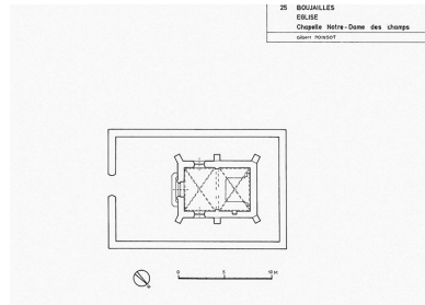
Plan au sol : relevé- croquis G. Poinso, 1975. Phot. Dominique et Sancey Dominguez IVR43_19792500005V
