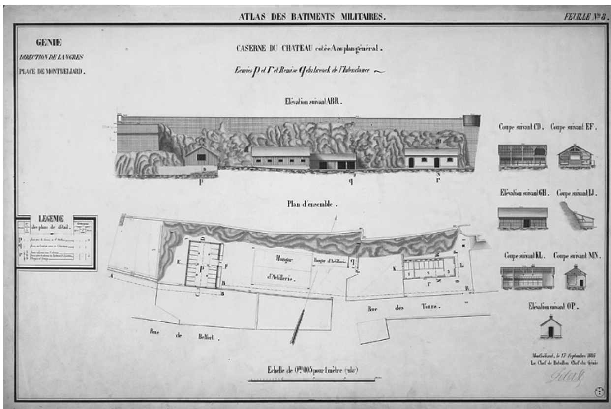
Caserne du château cotée A au plan général. Ecuries P et R et remise Q du break de l'Intendance [plans, coupes, élévations], 1886.
