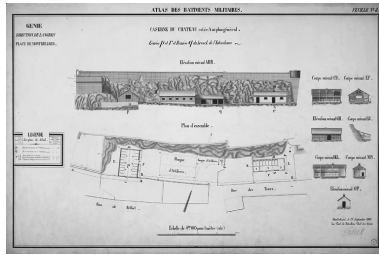
Caserne du château cotée A au plan général. Ecuries P et R et remise Q du break de l'Intendance [plans, coupes, élévations], 1886. Phot. Yves Sancey, Autr. Perlet IVR43_19862500217V
