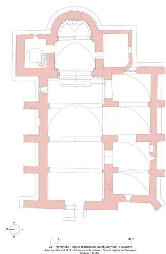
Plan de l'église. Dess. Alain Morelière IVR26_20132100057NUDA
