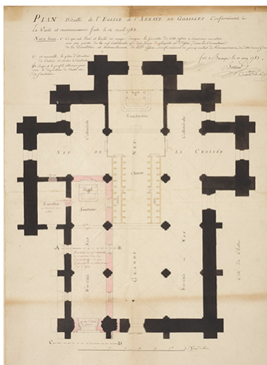
Plan détaillé de l'église de l'abbaye de Goailles, 1783. IVR43_20253900014NUC4A
