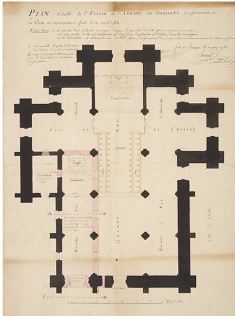
Plan détaillé de l'église de l'abbaye de Goailles, 1783.
