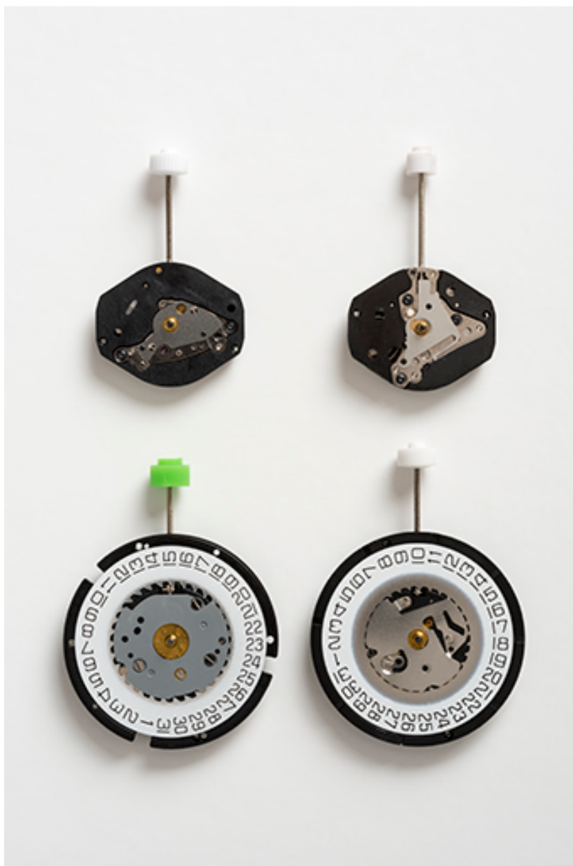
Vue d'ensemble des 4 mouvements : face côté cadran. De gauche à droite et de haut en bas : Isa 2326 et K 63, 317 et 2321.
