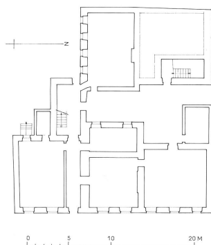
plan du rez-de-chaussée Dess. Jean-François Collin, Dess. Alain Morelière IVR26_20128900166A2YY
