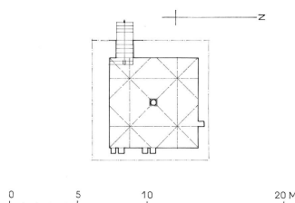
plan de cave Dess. Jean-François Collin, Dess. Alain Morelière IVR26_20128900167A4YY
