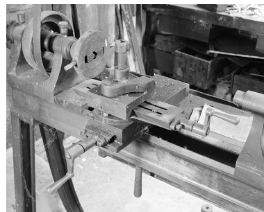
Le traînard entre la poupée fixe et la poupée mobile.
