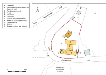
Plan-masse et de situation. Extrait du plan cadastral, 2015, section ZI. Dess. Mathias Papigny
