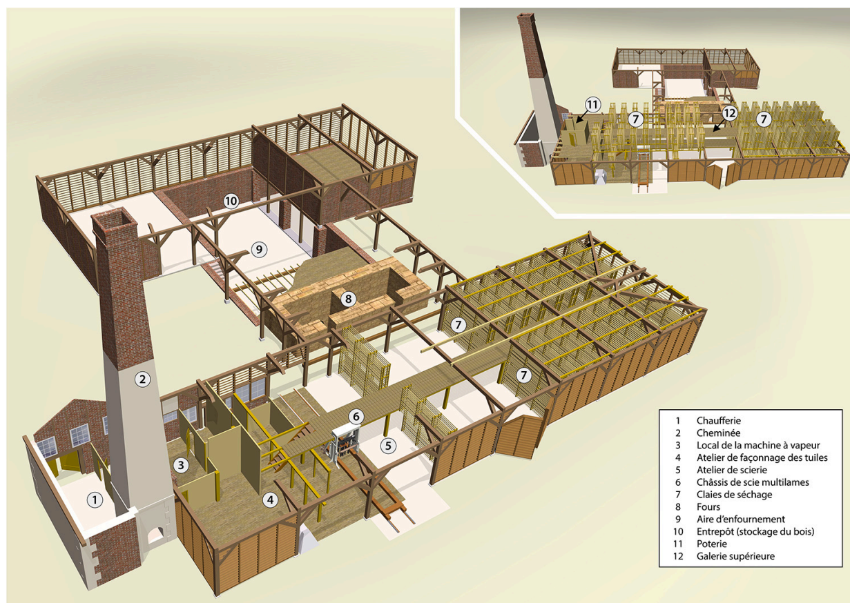
Vue axonométrique de la tuilerie-scierie.
