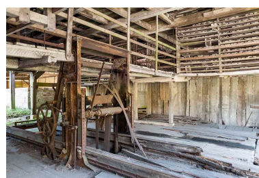
Châssis de scie et claies de séchage. Phot. Jérôme Mongreville IVR43_20152501081NUC4A
