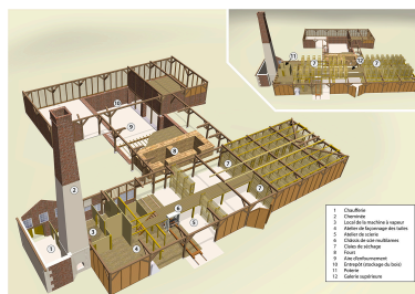
Vue axonométrique de la tuilerie-scierie. Dess. Mathias Papigny
