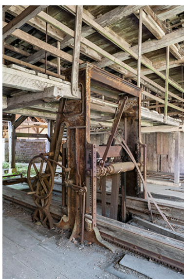
Châssis de scie à lames multiples Phot. Jérôme Mongreville IVR43_20152501080NUC4A
