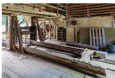
Châssis de scie et son chariot à grumes. Phot. Jérôme Mongreville IVR43_20152501889NUC4A
