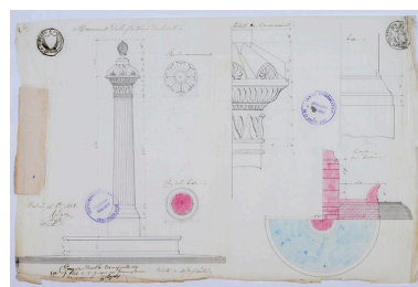
détails fontaine "du haut" Phot. , Autr. Jean-Baptiste Ridoux IVR43_20167001579NUC4A
