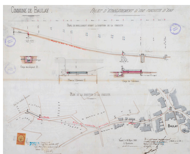
Projet d'établissement d'une conduite d'eau au Nord du village, passant par l'abreuvoir rue de Tallefosse et aboutissant au lavoir, place de la mairie, 1885 Phot. , Autr. Charles Desgranges IVR43_20167001578NUC4A
