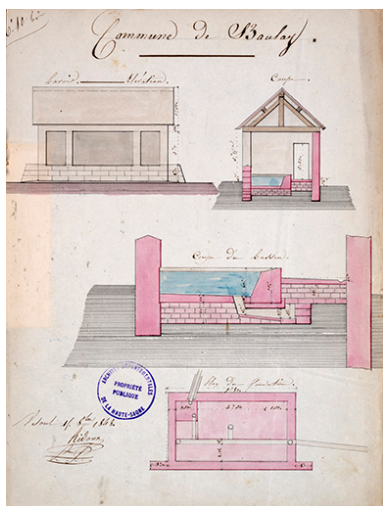
plans du lavoir aujourd'hui disparu Phot. , Autr. Jean-Baptiste Ridoux IVR43_20167001572NUC4A
