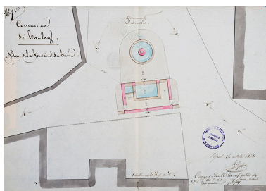
Plan de situation de la "fontaine du haut" du village, face au lavoir, 1848 Phot. , Autr. Jean-Baptiste Ridoux IVR43_20167001576NUC4A
