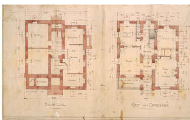
Villa L.N. Gauthier à Molinges [détails : plans du sous- sol et du rez-de-chaussée]. Phot. Jérôme Mongreville, Phot. Marius David IVR43_19973900059XA
