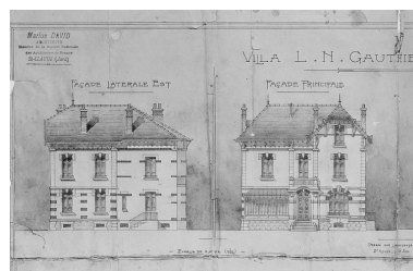
Villa L.N. Gauthier à Molinges [détails : façades antérieure et latérale droite]. Phot. Jérôme Mongreville, Phot. Marius David IVR43_19973900054X
