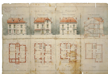
Villa L.N. Gauthier à Molinges. Phot. Jérôme Mongreville, Autr. Marius David IVR43_19973900053VA
