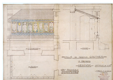
Villa de monsieur Gauthier à Molinges. Véranda. Détails au 1/20ème. Phot. Jérôme Mongreville, Phot. Marius David IVR43_19973900050VA
