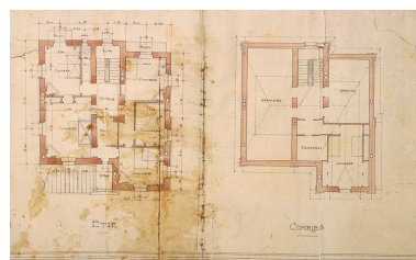
Villa L.N. Gauthier à Molinges [détails : plans de l'étage et du comble]. Phot. Jérôme Mongreville, Phot. Marius David IVR43_19973900061XA
