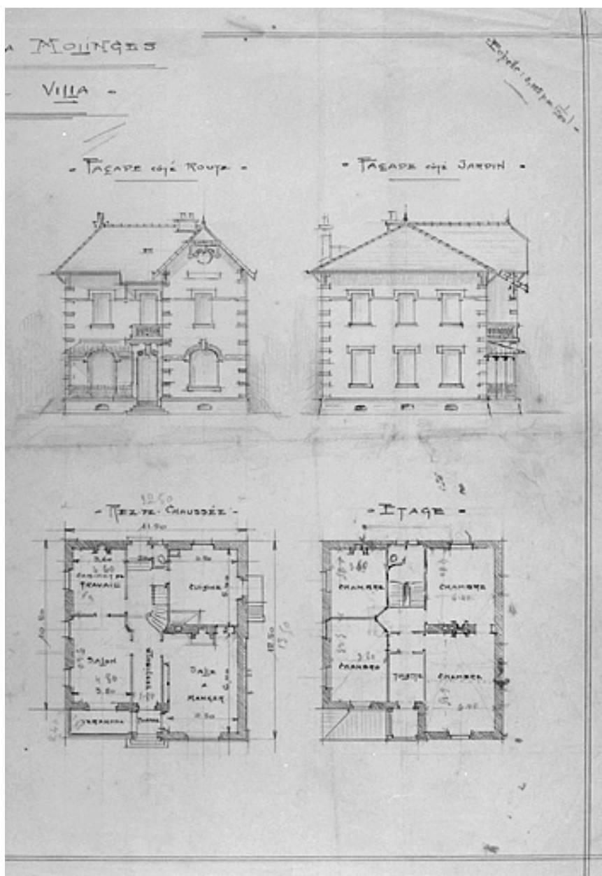
M. N. Gauthier à Molinges. Avant-projets de Villa [détail de la partie droite : 2e avant-projet].
