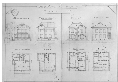
M. N. Gauthier à Molinges. Avant-projets de Villa. Phot. Jérôme Mongreville, Phot. Marius David IVR43_19973900051V
