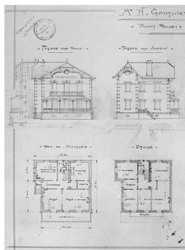
M. N. Gauthier à Molinges. Avant-projets de Villa [détail de la partie gauche : 1er avant-projet]. Phot. Jérôme Mongreville, Phot. Marius David IVR43_19973900067X
