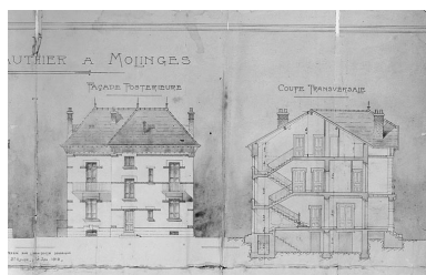
Villa L.N. Gauthier à Molinges [détails : façade postérieure et coupe]. Phot. Jérôme Mongreville, Phot. Marius David IVR43_19973900056X
