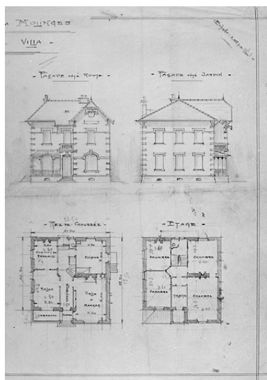
M. N. Gauthier à Molinges. Avant-projets de Villa [détail de la partie droite : 2e avant-projet]. Phot. Jérôme Mongreville, Phot. Marius David IVR43_19973900066X
