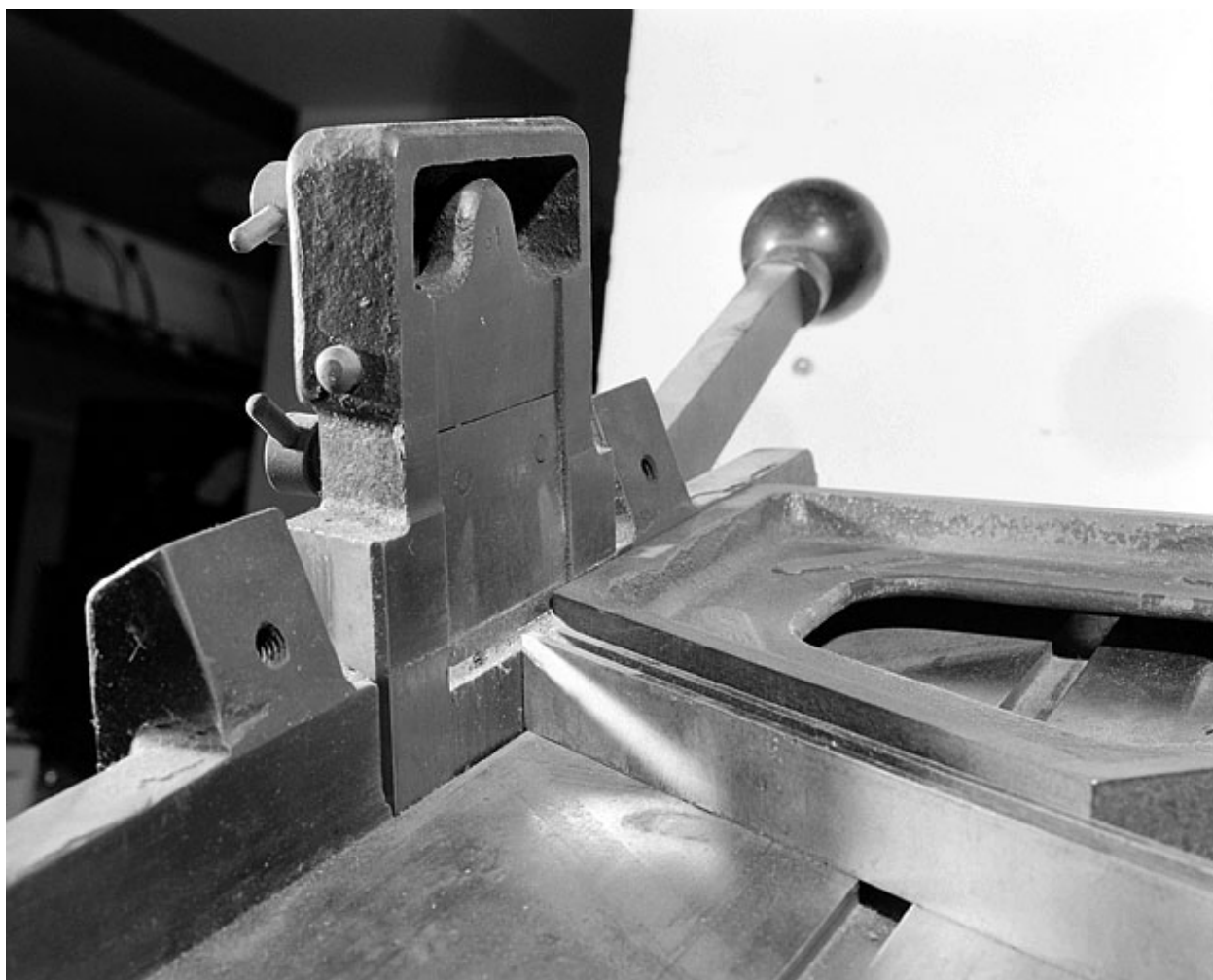
Coupe oblique d'un filet avec le "couteau-rabot". Le filet est appuyé contre le guide pentagonal.
