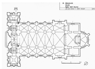
Plan au sol : relevé-croquis J.M. Demoly et G. Poinso, 1975. Phot. Dominique et Sancey Dominguez IVR43_19792500001V
