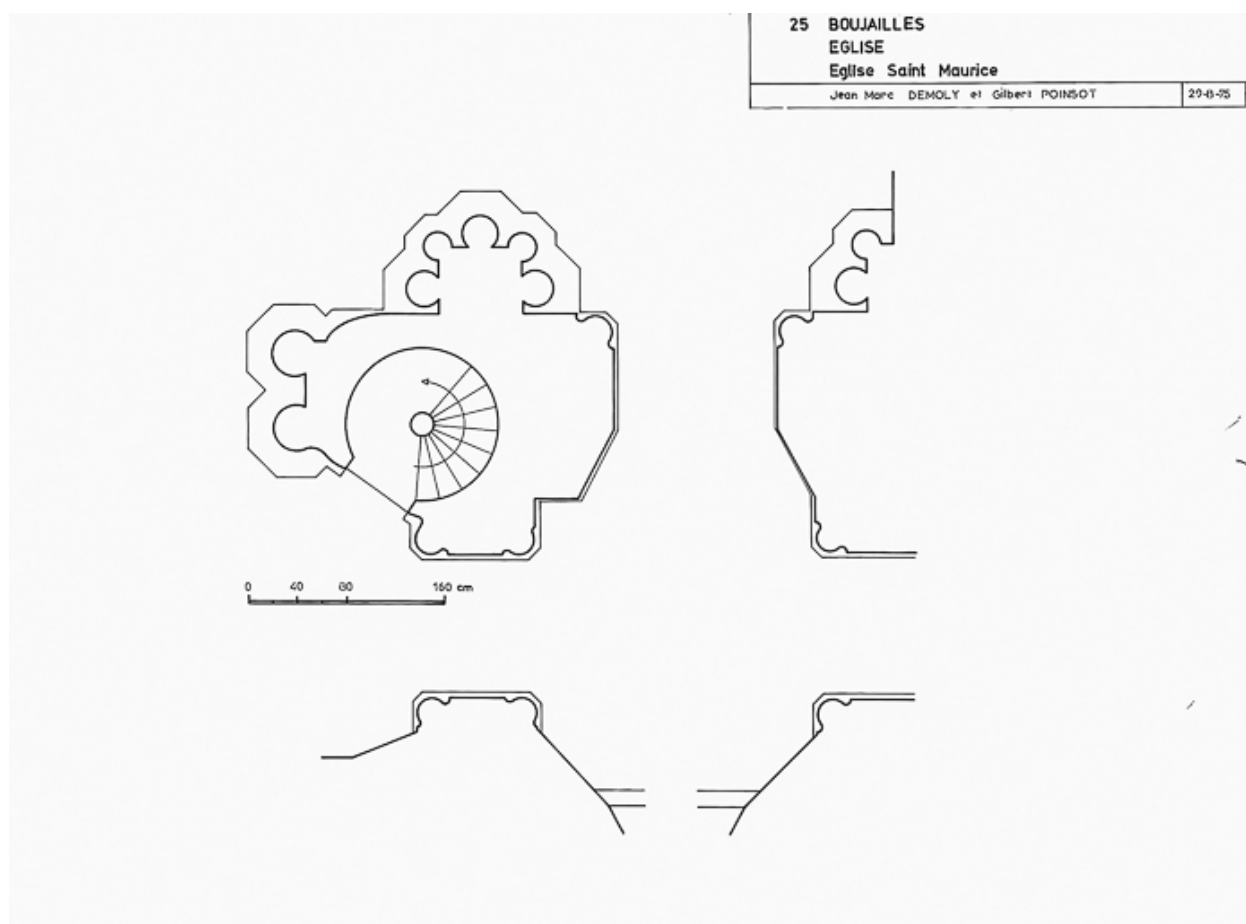
Plan des piliers d'entrée : relevé-croquis J.M Demoly et G. Poinot, 1975.
