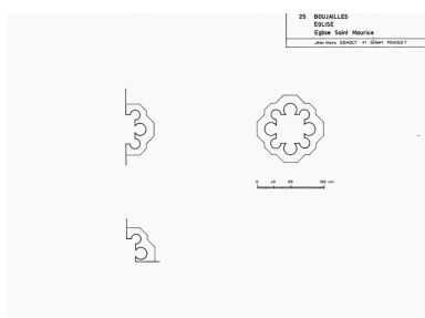
Plan des petits piliers : relevé-croquis J.M. Demoly et G. Poinso, 1975. Phot. Dominique et Sancey Dominguez IVR43_19792500003V
