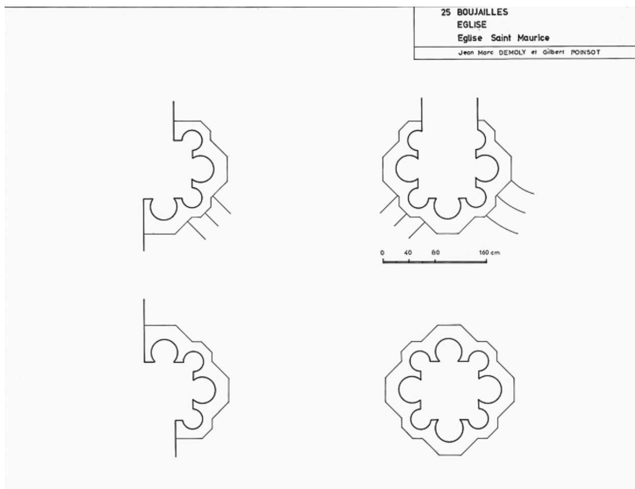
Plan des gros piliers : relevé-croquis J.M Demoly et G. Poinso, 1975.
