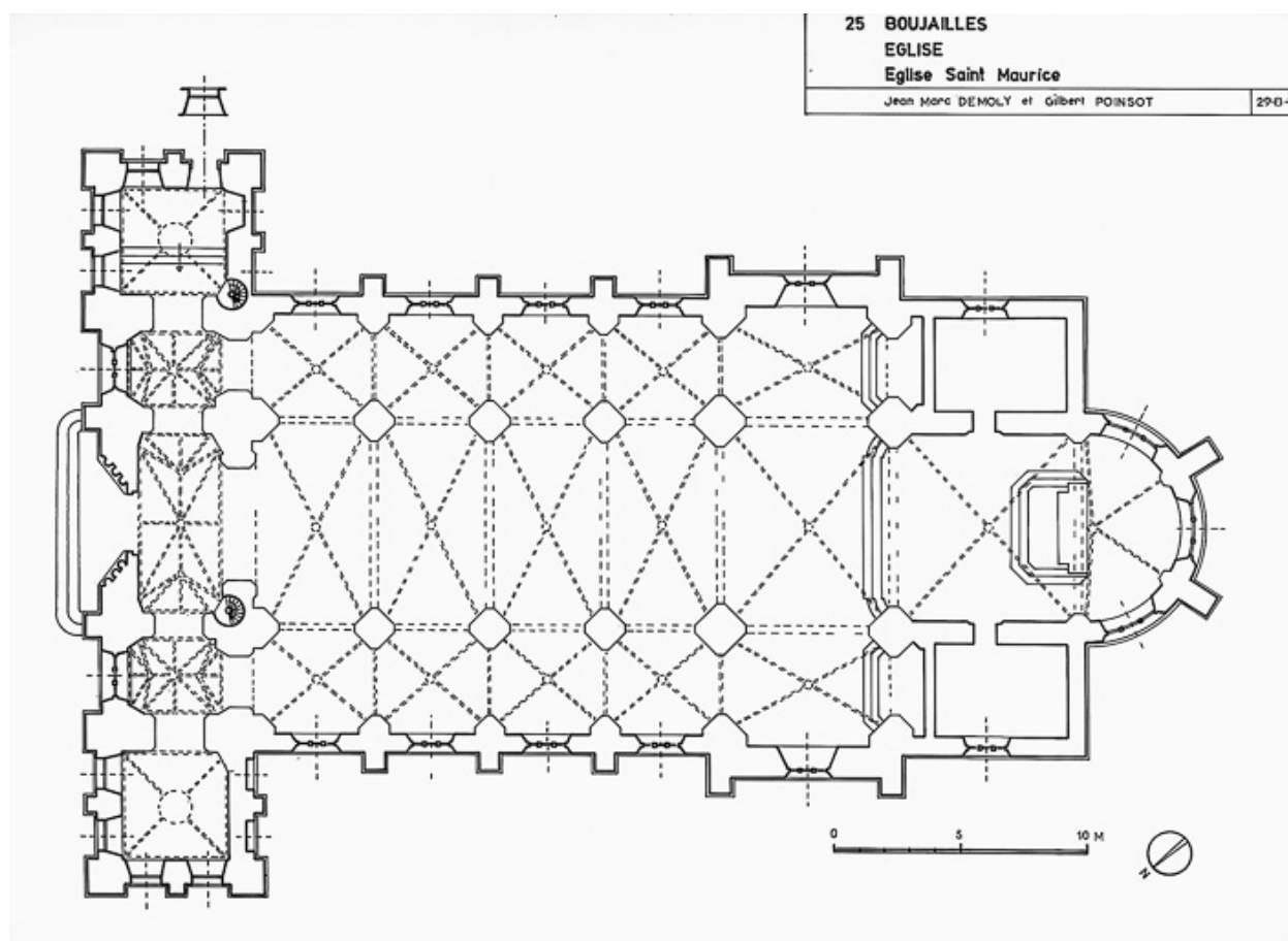
Plan au sol : relevé-croquis J.M. Demoly et G. Poinot, 1975.
