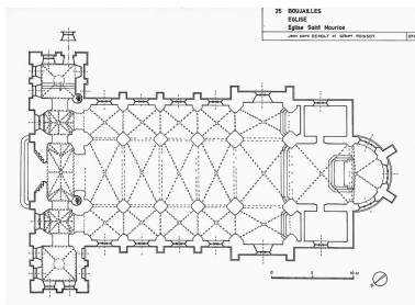
Plan au sol : relevé-croquis J.-M. Demoly et Gilbert Poinso, 1975. Phot. Dominique et Sancey Dominguez IVR43_19792500001V
