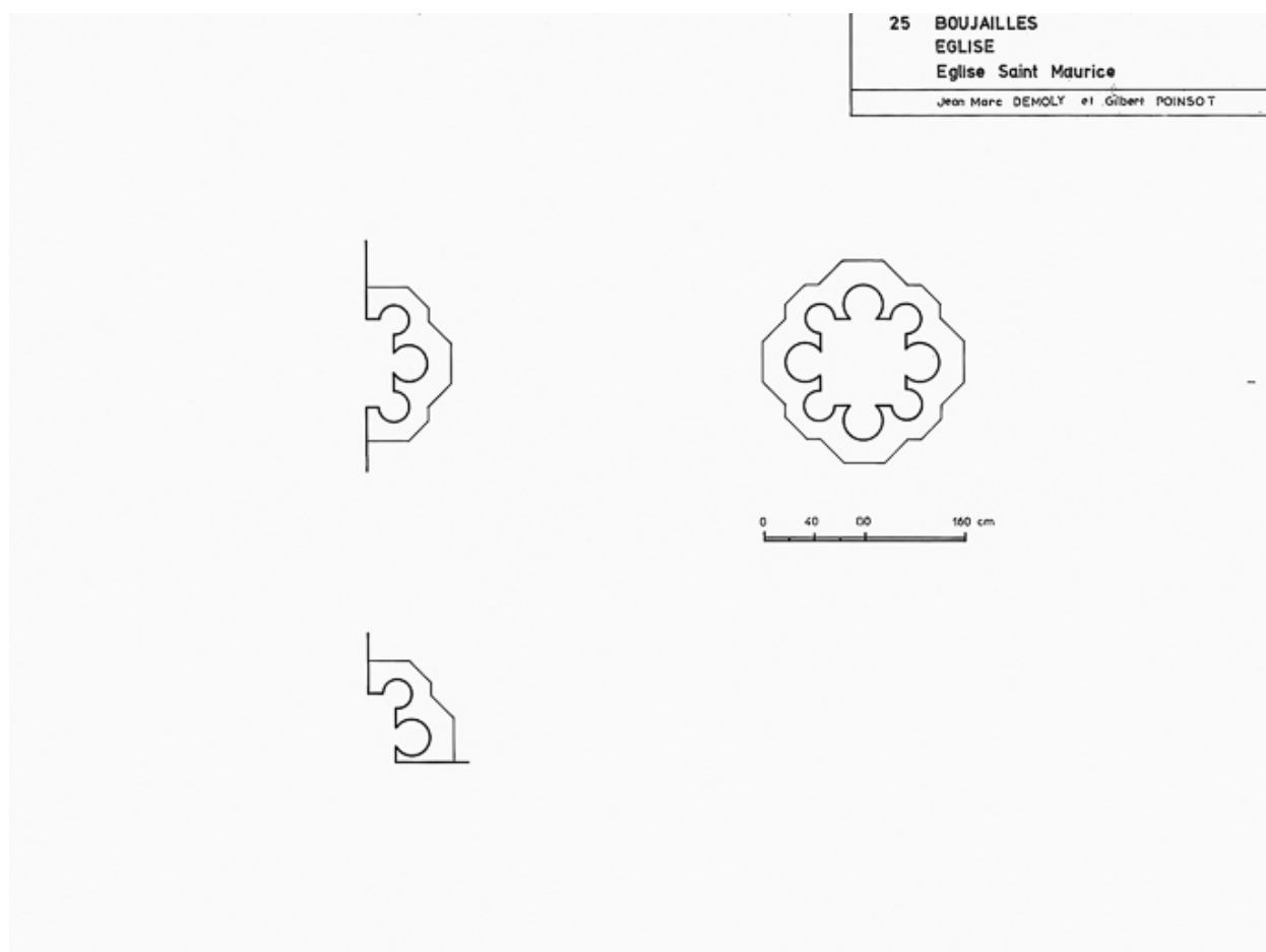
Plan des petits pilliers : relevé-croquis J.M. Demoly et G. Poinsoy, 1975.
