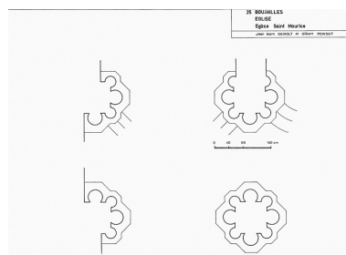
Plan des gros piliers : relevé-croquis J.M Demoly et G. Poinso, 1975. Phot. Dominique et Sancey Dominguez IVR43_19792500004V
