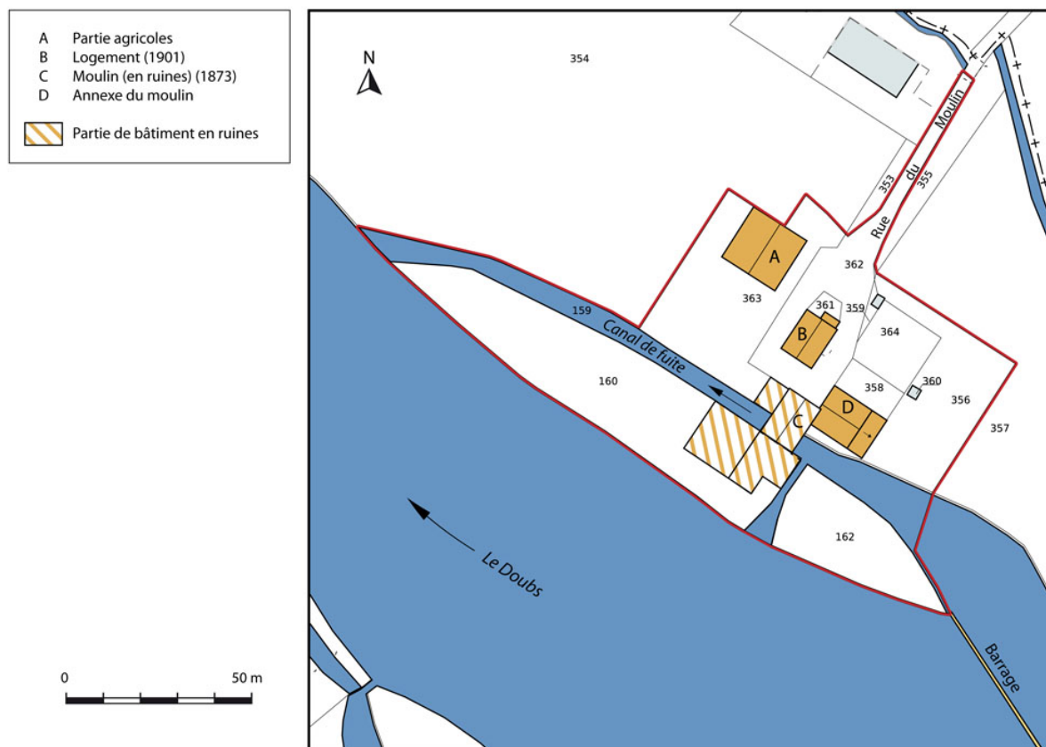
Plan-masse et de situation. Extrait du plan cadastral numérisé, section A, échelle 1:1000.
