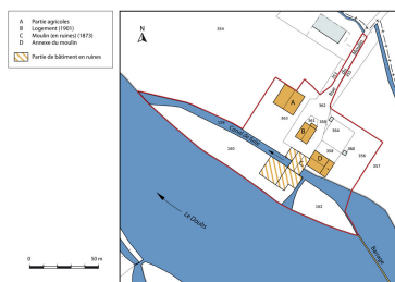
Plan-masse et de situation. Extrait du plan cadastral numérisé, section A, échelle 1:1000. Dess. Mathias Papigny IVR43_20142500567NUDA
