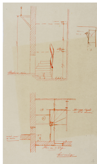
[Croquis de plan et coupe de l'escalier pour le concierge]. S.d. [1898 ?]. Phot. Pierre-Marie Barbe-Richaud, Autr. Charles Brazeau IVR26_20245800436NUC2A
