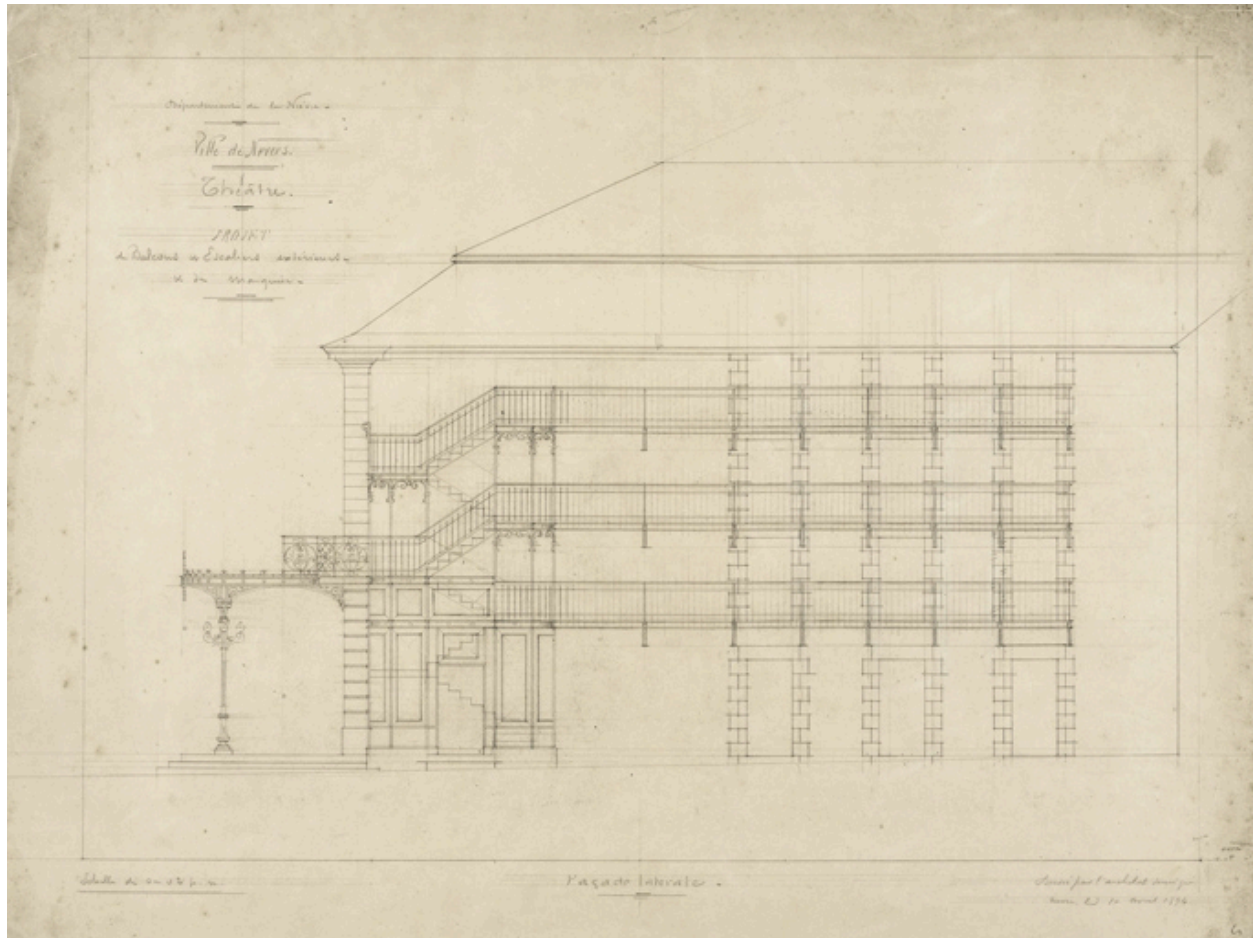
Ville de Nevers. Théâtre. Projet de balcons et escaliers extérieurs et de marquise. Façade latérale. 10 avril 1894.
