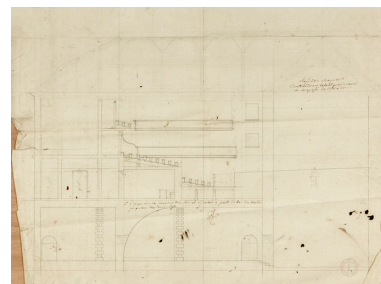
[Projet de salle de spectacle : plans et coupe]. N° 5 Coupe sur la longueur de la salle de spectacle à partir du bas des voûtes jusqu'au deuxième étage. S.d. [1809 ?]. Phot. Pierre-Marie Barbe-Richaud IVR26_20245800455NUC2A
