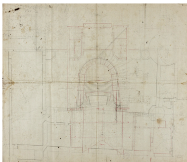
[Projet de salle de spectacle : plans et coupe]. N° 3 Plan des premières loges et des parties latérales pour le logement des acteurs et pour le magasin des décorations. S.d. [1809 ?]. Phot. Pierre-Marie Barbe-Richaud IVR26_20245800465NUC2A
