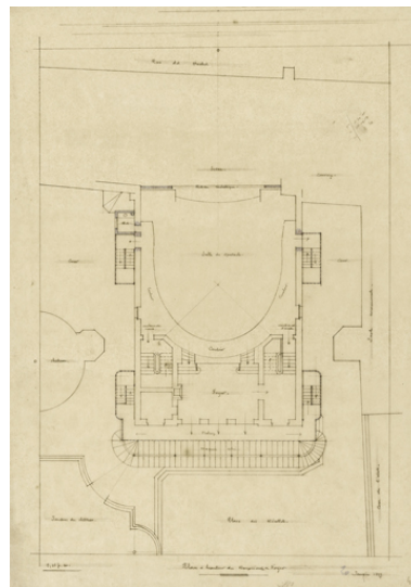
Théâtre. Projet de marquise vitrée et d'escaliers extérieurs. Plan à hauteur des Deuxièmes et Foyer. 20 janvier 1897.
