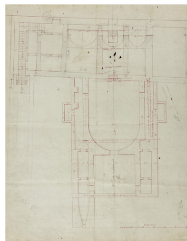
[Projet de salle de spectacle : plans et coupe]. N° 1er Plan des fondements. S.d. [1809 ?]. Phot. Pierre-Marie Barbe-Richaud IVR26_20245800462NUC2A
