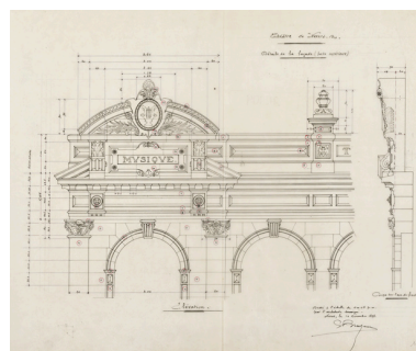
Théâtre de Nevers. Détails de la façade (partie supérieure). 10 décembre 1898.
