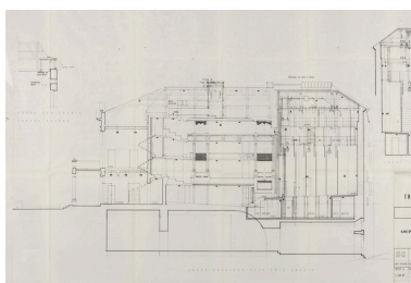
Ville de Nevers. Théâtre municipal. Mise en conformité. 6B. Coupe longitudinale. 1976. Phot. Pierre-Marie Barbe-Richaud, Autr. Camille Demangeat, Autr. Michel Rioualec IVR26_20245800469NUC4A
