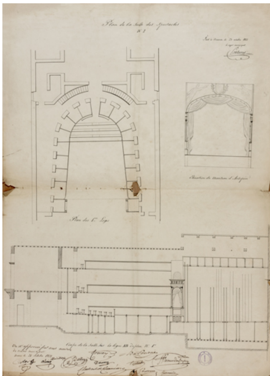
Plan de la salle des spectacles. N° 2. Plan des 1ères loges, Coupe de la salle sur la ligne AB du plan N° 1er [et] Elévation du Manteau d'Arlequin. 23 octobre 1822.
