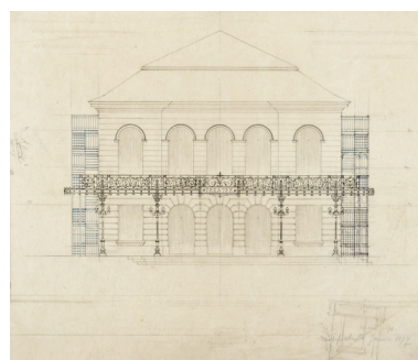
[Projet de façade avec marquise et escaliers latéraux]. 10 avril 1894 modifié le 20 janvier 1897. Phot. Pierre-Marie Barbe- Richaud, Autr. Charles Brazeau IVR26_20245800420NUC2A
