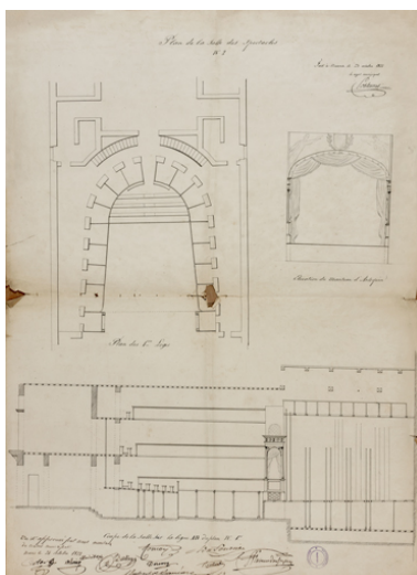
[Projet de salle de spectacle : plans et coupe]. N° 3 Plan des premières loges et des parties latérales pour le logement des acteurs et pour le magasin des décorations. S.d. [1809 ?]. Phot. Pierre-Marie Barbe-Richaud IVR26_20245800465NUC2A
