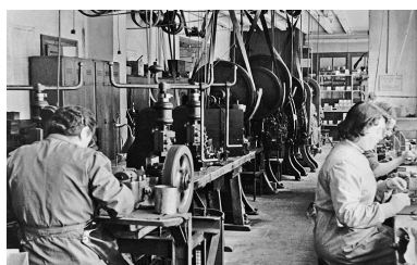
Atelier des apprêts : fabrication de composants de lunettes. Photographie, 1958. Phot. Jérôme Mongreville IVR43_19913900284X
