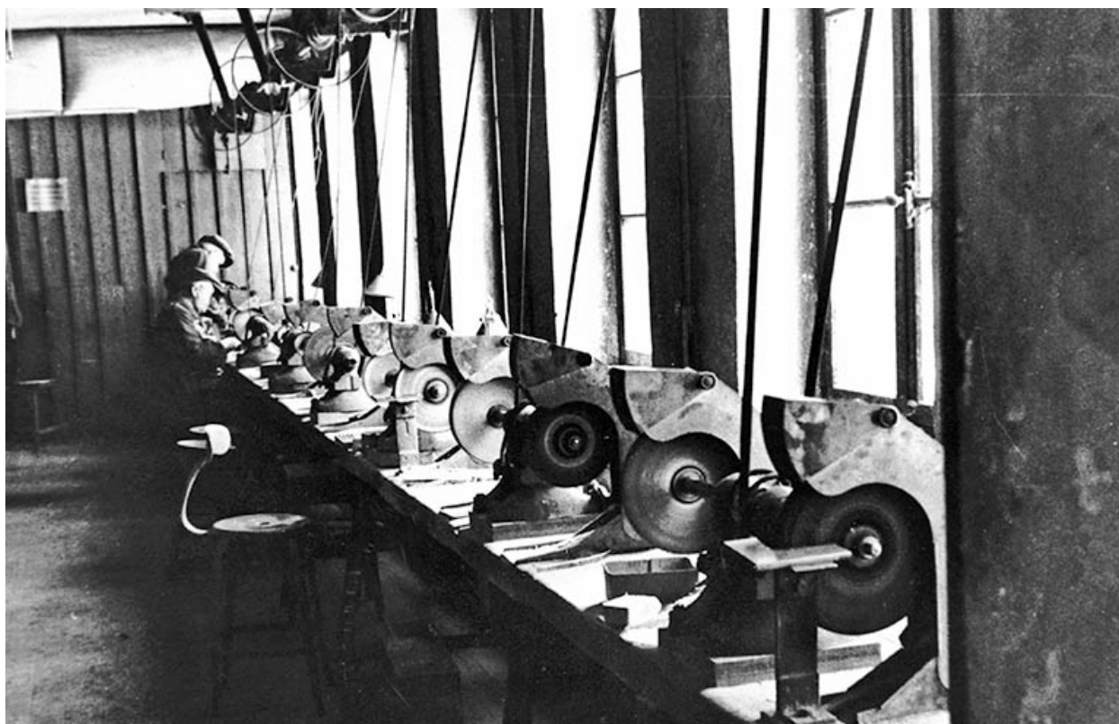
Polissage des lunettes au tampon. Photographie, 1958.
