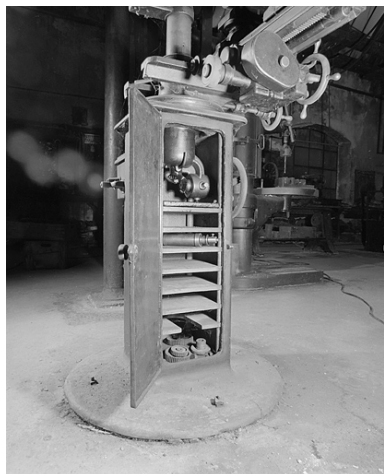
Détail du double système de commande manuelle.
