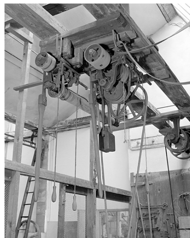
Détail du double système de transmission. Phot. Yves Sancey IVR43_20022500862X
