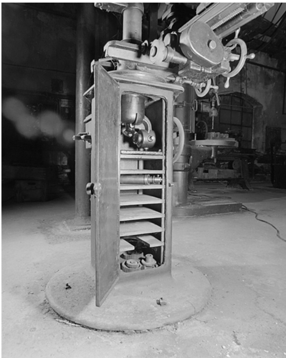
Détail du double système de commande manuelle.
