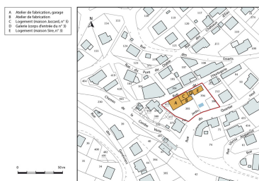
Plan-masse et de situation. Dess. Mathias Papigny IVR43_20162501525NUDA
