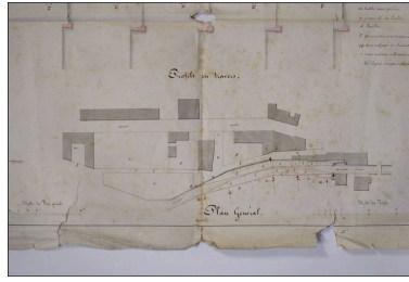
Projet pour le redressement du lit de la rivière et l'agrandissement du quai de la Promenade, 1843. Phot. Yves Sancey, Phot. Vital Ponard IVR43_20103900076NUC2A
