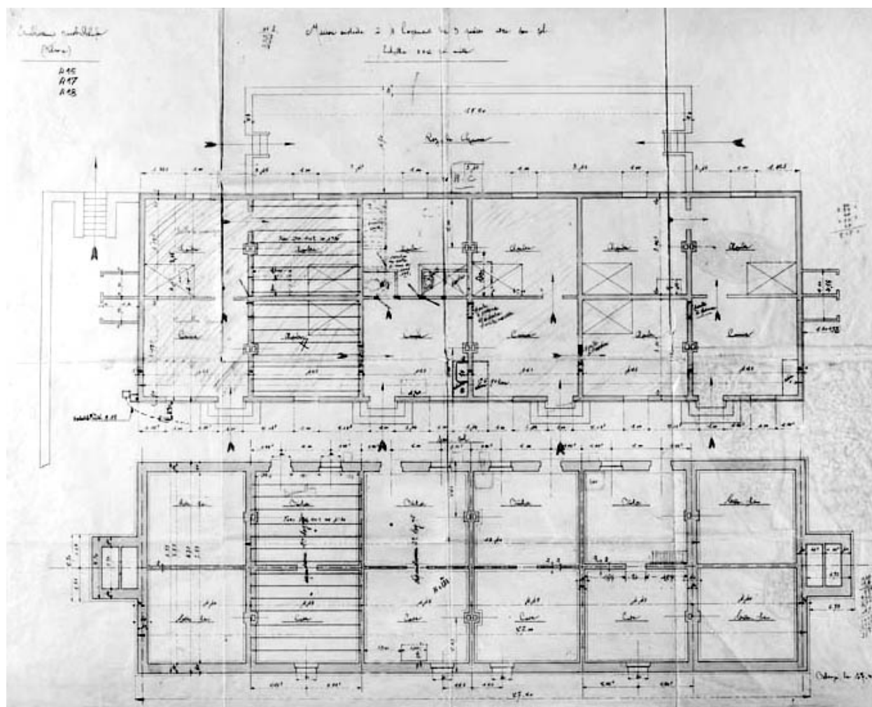
Etablissement Jacob-Delafor (Belvoje). Maison ouvrière à 4 logements de 3 pièces avec sous-sol.
