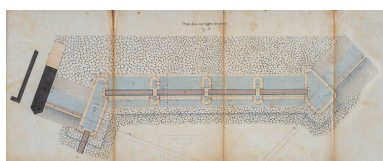
Achèvement du bief de Vereux - Exhaussement du barrage de Vereux (1881) : plan des ouvrages projetés. Phot. Jérôme Mongreville, Autr. Gustave Bouvaist IVR43_20207000178NUC4A
