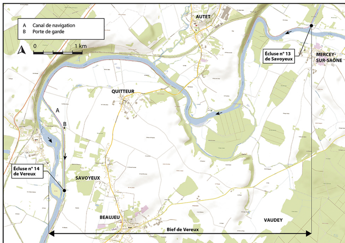
Plan de localisation (1/25 000). Extrait du ScanExpress standard © IGN 2018.
