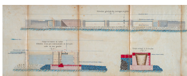
Achèvement du bief de Vereux - Exhaussement du barrage de Vereux (1881) : élévation générale des ouvrages projetés. Phot. Jérôme Mongreville, Autr. Gustave Bouvaist IVR43_20207000179NUC4A
