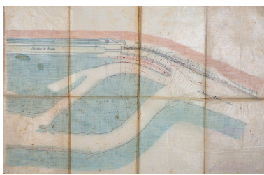
Achèvement du bief de Vereux - Digue de Vereux (1881). Phot. Jérôme Mongreville, Autr. Gustave Bouvaist IVR43_20207000176NUC4A
