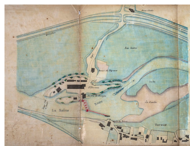
Achèvement du bief de Vereux - Exhaussement du barrage de Vereux (1881) : plan général. Phot. Jérôme Mongreville, Autr. Gustave Bouvaist IVR43_20207000177NUC4A
