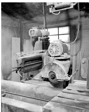
Débiteuse-mouleuse sud : bâti vertical, moteur et toupie. Phot. Yves Sancey IVR43_19933900345X
