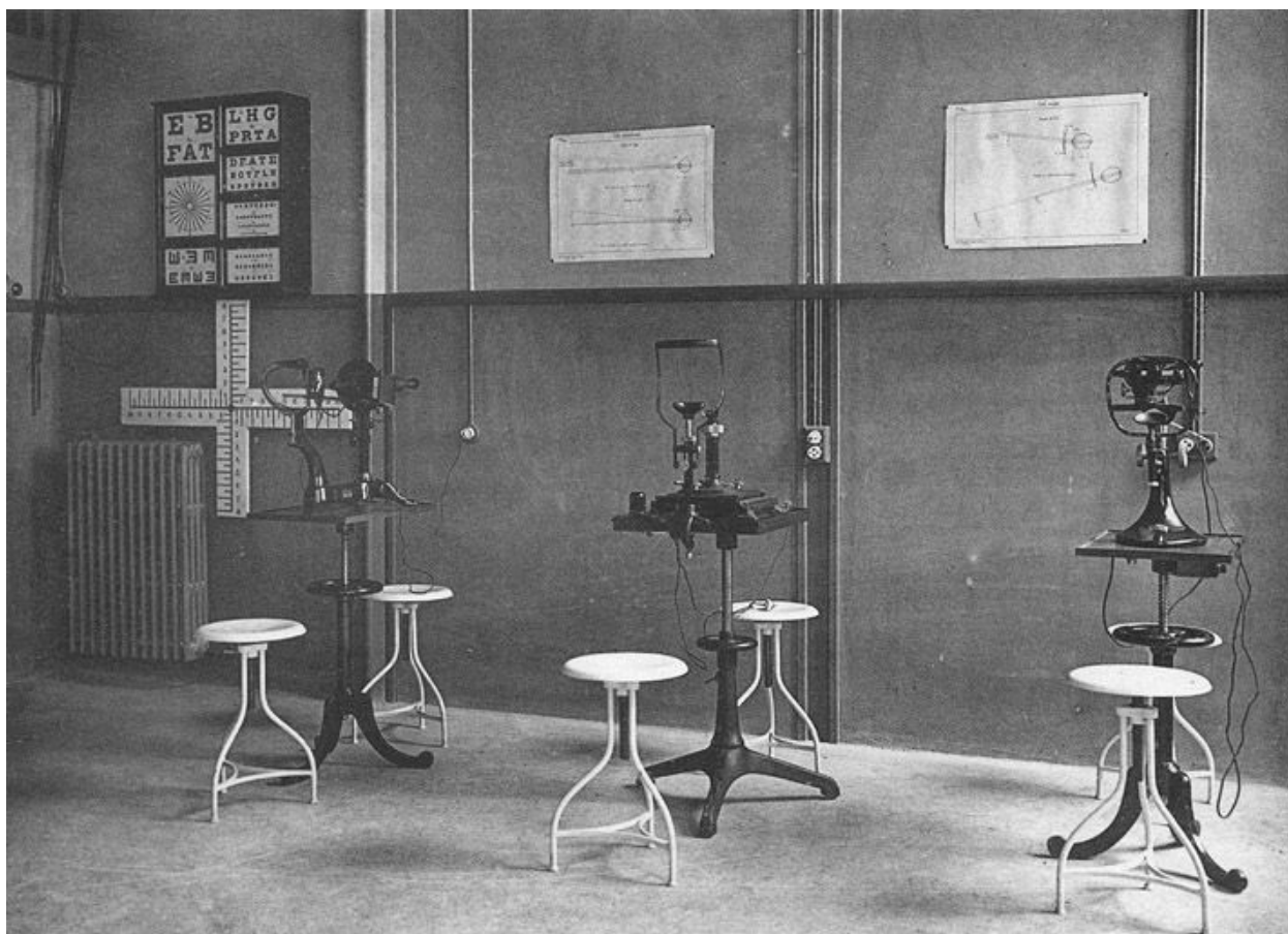
Laboratoire d'Optométrie, décennies 1930-1940. Réfracteur à gauche, lampe à fente à droite.
