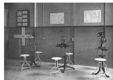
Laboratoire d'Optométrie, décennies 1930-1940. Réfracteur à gauche, lampe à fente à droite. Phot. Yves Sancey, Autr. David J. et Vallois E. (Ets) IVR43_20103900694NUC2A
