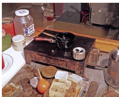
Chaufettere pour le polissoir à poix. Bâtiment de l'enseignement (F), atelier de fabrication des composants optiques. Déposée à la surface de l'outil, la poix en épouse la forme et use le composant via un produit abrasif intercalé entre eux. Phot. Jérôme Mongreville IVR43_20033901029XA
