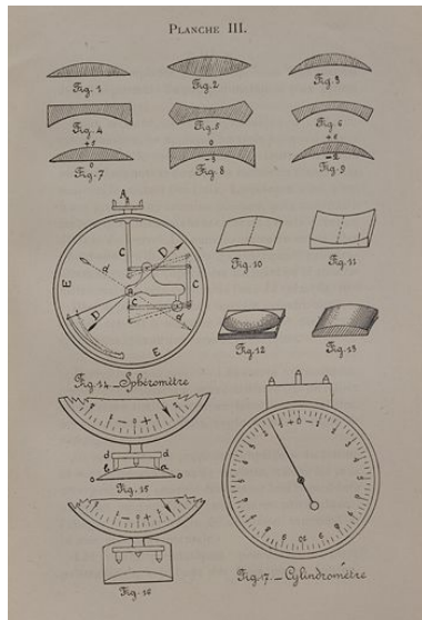
Verres sphériques, verres cylindriques [et] Instruments de mesure, 1913 Phot. Yves Sancey, Autr. Léon Emard IVR43_20093900053NUC2A
