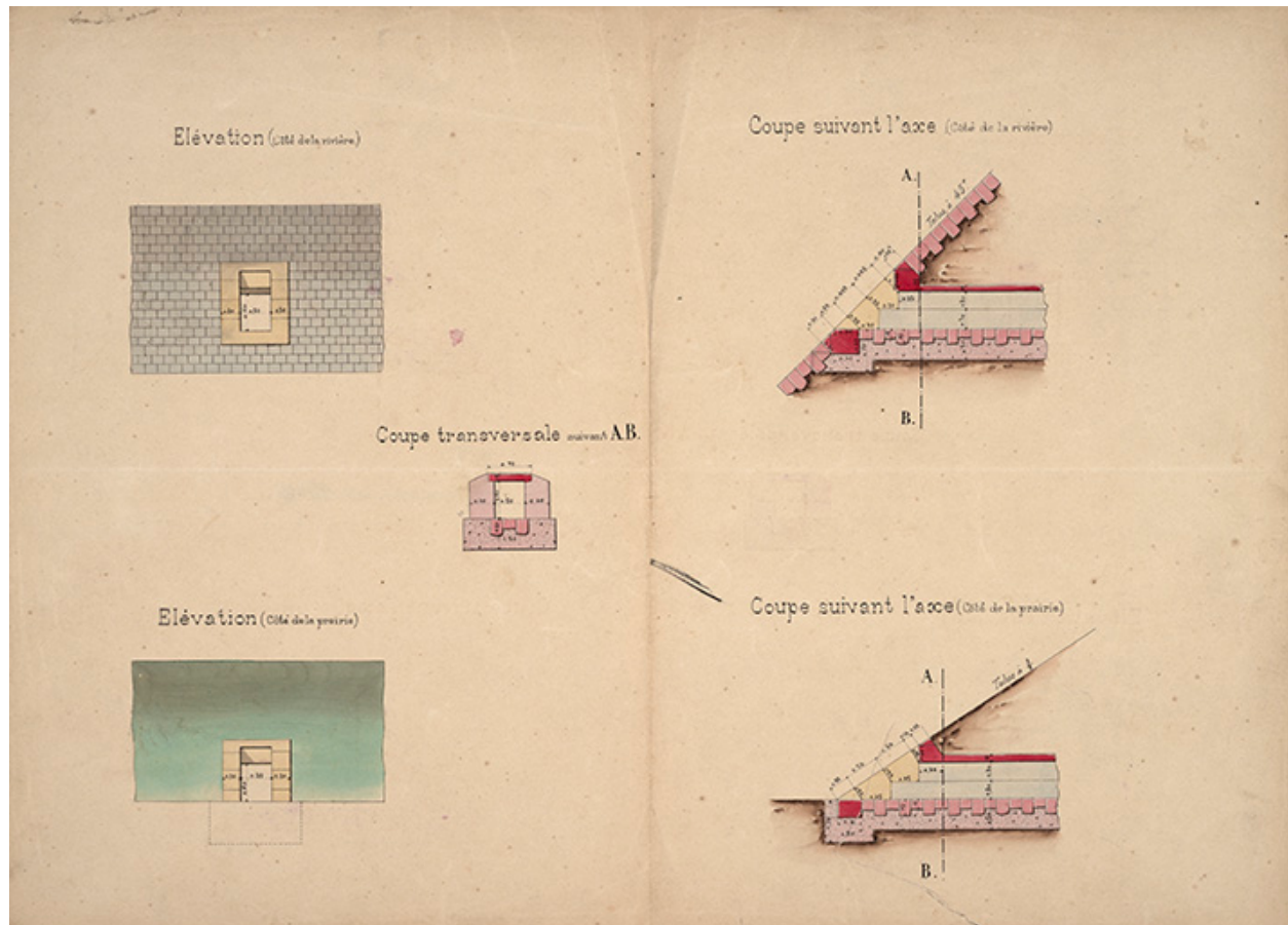
Dérivation de Chemilly - Type des aqueducs (1878).
