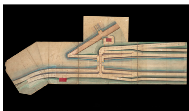
Plan des abords de la porte de garde (1878). Phot. Jérôme Mongreville, Autr. Gustave Bouvaist IVR43_20207000155NUC4A
