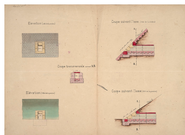
Dérivation de Chemilly - Type des aqueducs (1878). Phot. Jérôme Mongreville, Autr. Gustave Bouvaist IVR43_20207000156NUC4A
