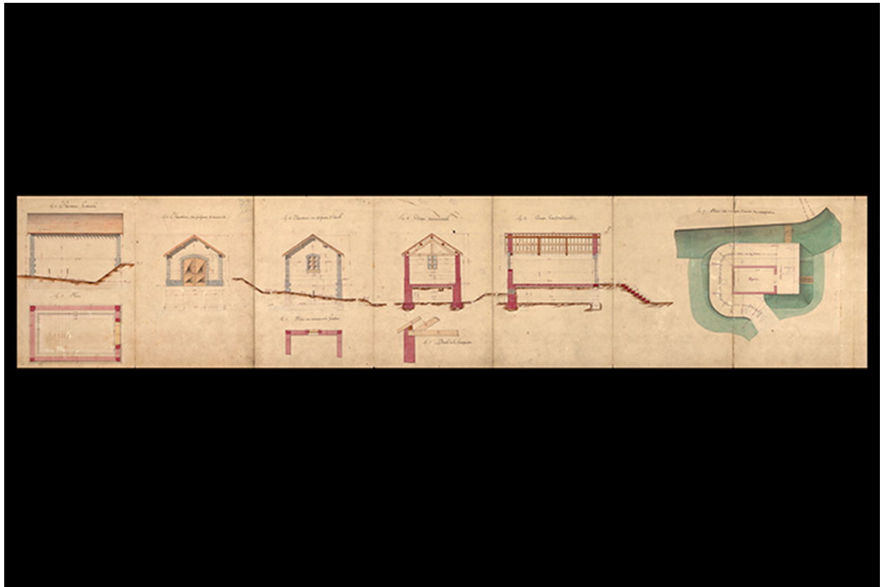
Dérivation de Chemilly - Magasin (1878).
