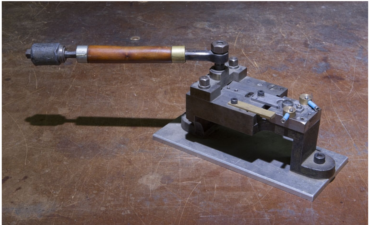
Machine à cintrer les nez, à coulisseau horizontal.
