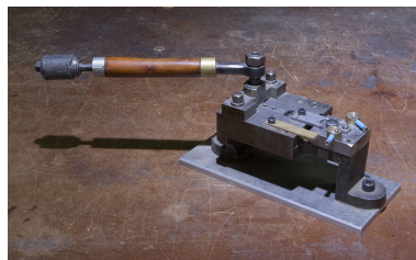
Machine à cintrer les nez, à coulisseau horizontal. Phot. Yves Sancey IVR43_20103900286NUC2A
