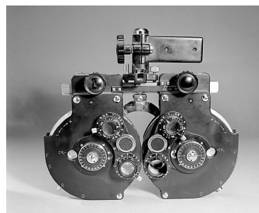
Deuxième phoroptère : face avant. Phot. Jérôme Mongreville IVR43_20023900240X
