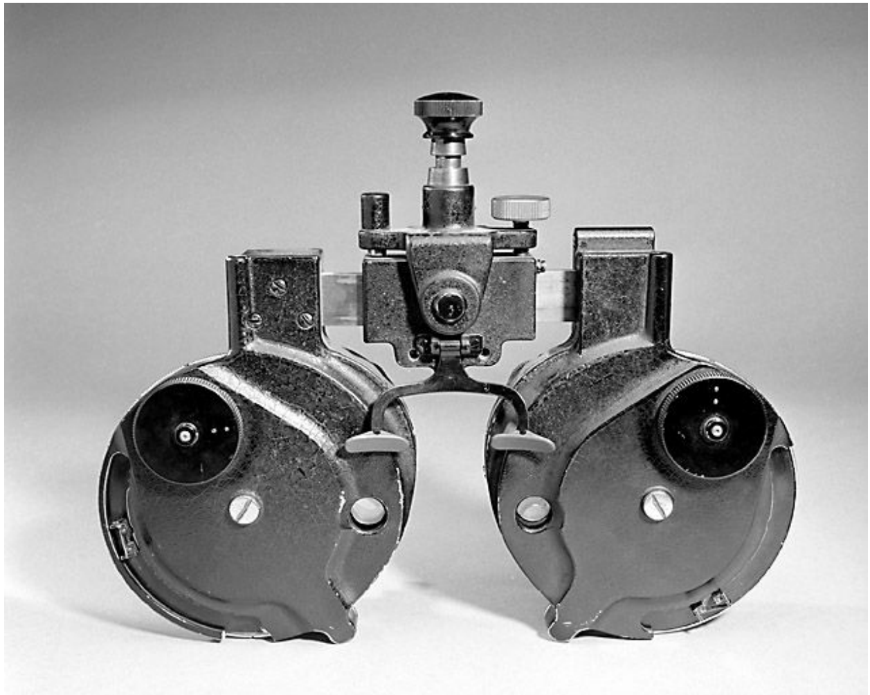
Premier phoroptère : face arrière.
