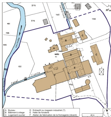
Plan-masse et de situation. Extrait de plan cadastral numérisé, 2008, section A, 1:1250 Source : Direction générale des Finances Publiques - Cadastre ; mise à jour : 2008. Dess. André Céréza IVR43_20087000488NUDA
