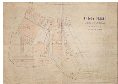
Ets Japy Frères. Usine du Rondelot - Plan général et conduite à vapeur. Plan, tirage, s.n., échelle 1/500, septembre 1935. Phot. Jérôme Mongreville IVR43_20122501176NUC4A
