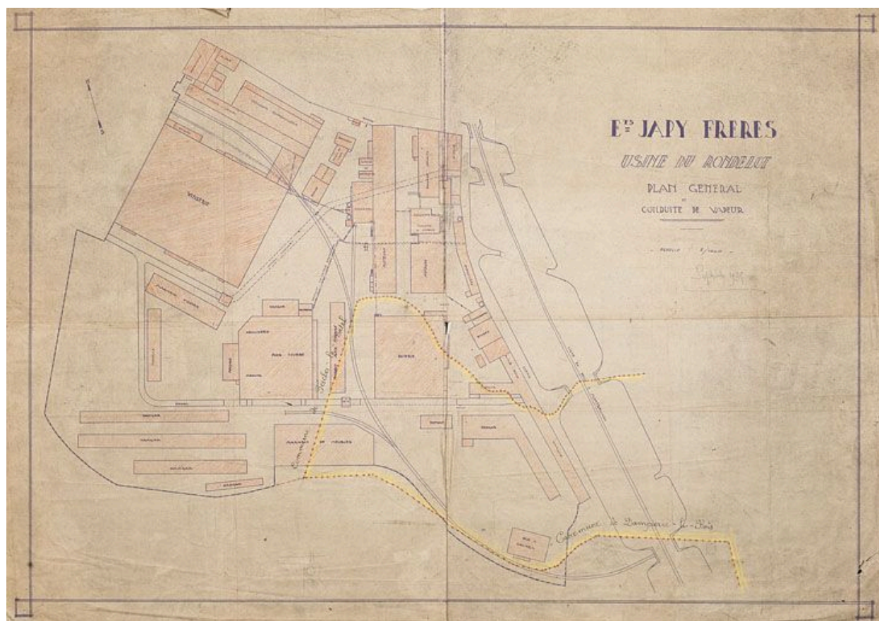
Ets Japy Frères. Usine du Rondelot - Plan général et conduite à vapeur. Plan, tirage, s.n., échelle 1/500, septembre 1935.
