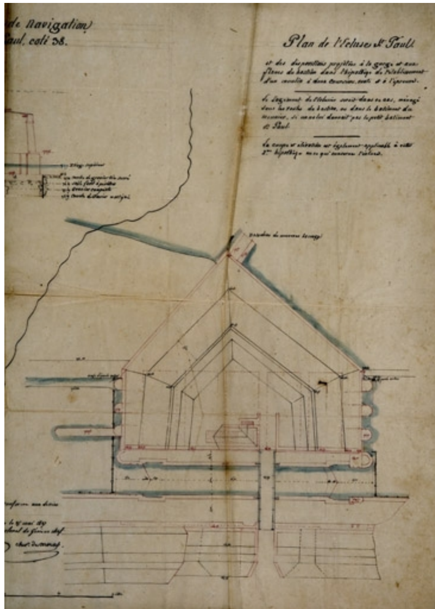
Plans et détails relatifs à l'écluse de navigation à établir à la gorge du bastion St Paul, coté 38 [détail], 1827.
