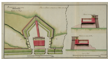
Besançon pour 1764. Plan et profils du bastion St Paul coté 20, 1764. Phot. Yves Sancey, Phot. Tanquerëyd IVR43_20062500367NUCA
