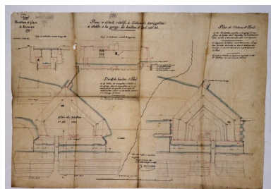
Plans et détails relatifs à l'écluse de navigation à établir à la gorge du bastion St Paul, coté 38 [plans, coupe et élévation], 1827. Phot. Yves Sancey IVR43_20062500362NUCA
