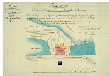
Plan du bastion de St Paul, coté 38 (au projet relatif au canal), et du moulin du même nom, avec ses dépendances [...], 1826. Phot. Yves Sancey, Phot. Picot de Moras IVR43_20062500074NUCA
