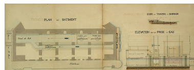
Règlement d'eau du moulin St Paul appartenant à l'administration de la Guerre. Dessin de détails [plan du bâtiment, coupe du barrage et élévation de la prise d'eau], 1874. Phot. Yves Sancey, Phot. Rascol IVR43_20062500093NUCA
