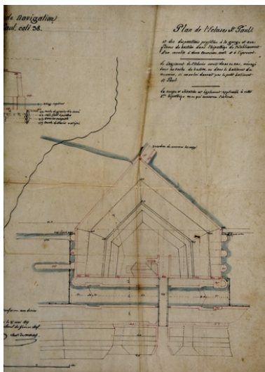
Plans et détails relatifs à l'écluse de navigation à établir à la gorge du bastion St Paul, coté 38 [détail], 1827. Phot. Yves Sancey IVR43_20062500363NUCA
