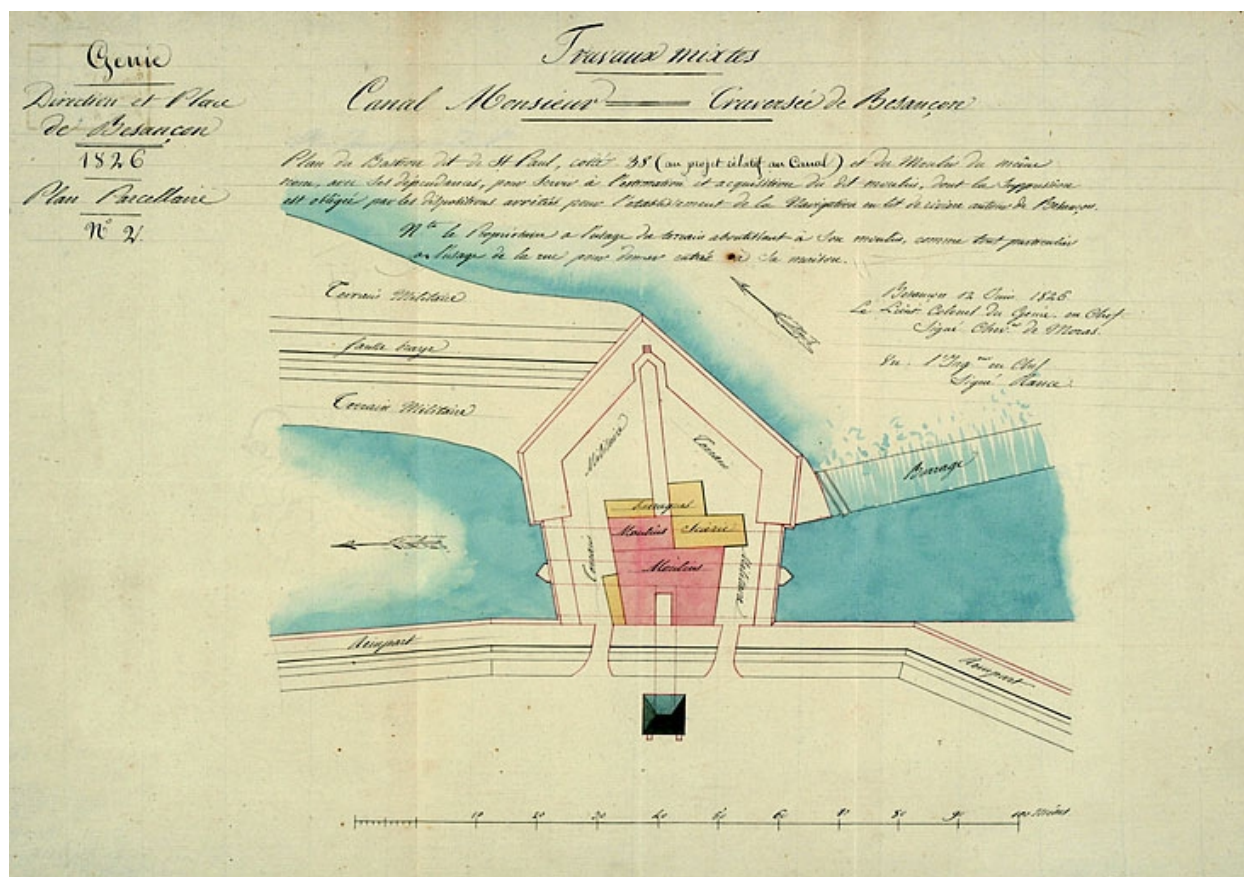
Plan du bastion de St Paul, côté 38 (au projet relatif au canal), et du moulin du même nom, avec ses dépendances [...], 1826.
