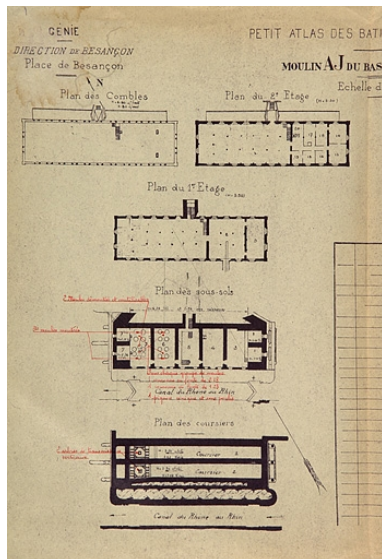
Petit atlas des bâtiments militaires. Moulin AJ du bastion St Paul [plans], 1938. Phot. Yves Sancey IVR43_20062500108NUCA
