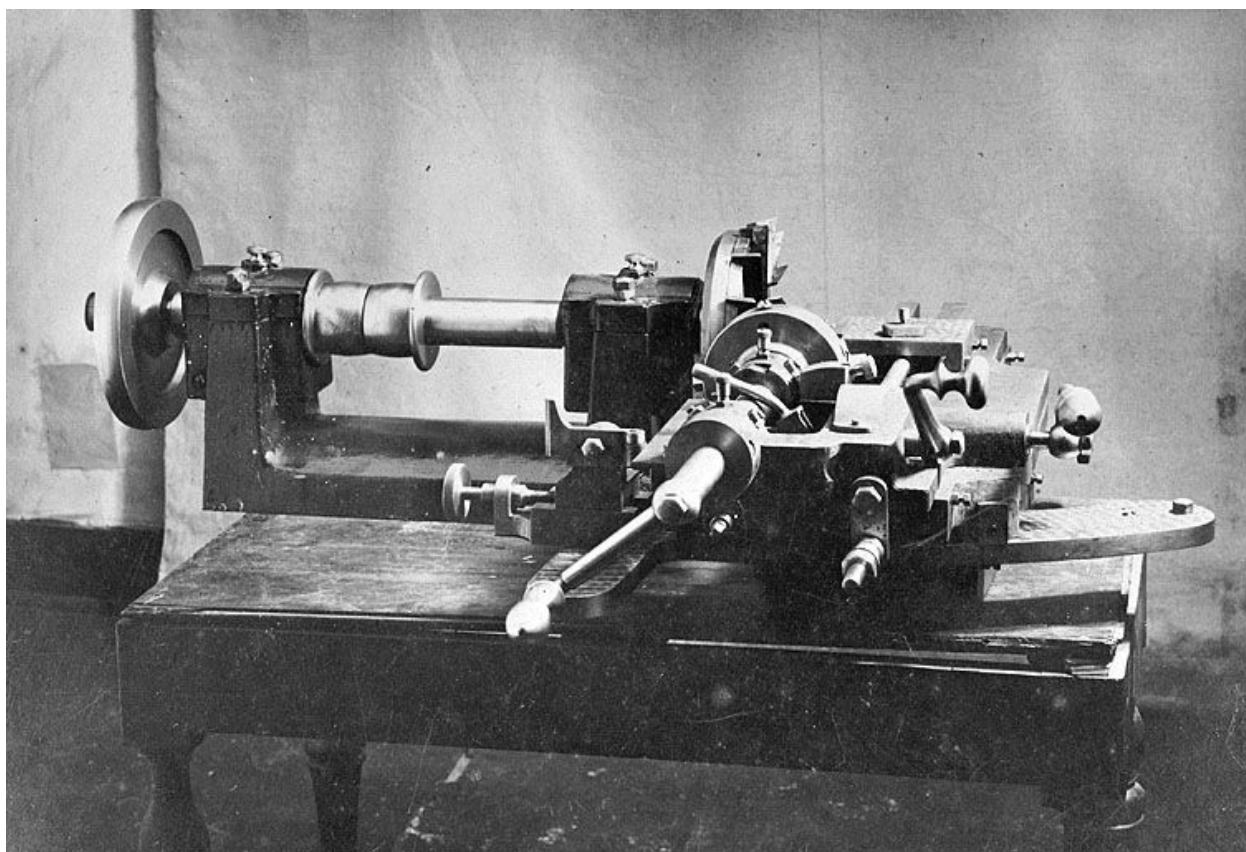
Exemple de machine à aplatir du constructeur mécanicien Lizon.
