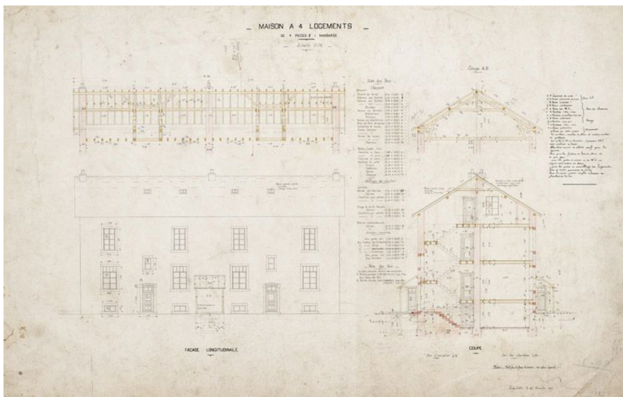
Maison à quatre logements de 4 pièces et une mansarde. Plan, encre, lavis, échelle 1/50, Lafeschotte, 26 novembre 1919.
