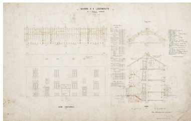
Maison à quatre logements de 4 pièces et une mansarde. Plan, encre, lavis, échelle 1/50, Lafeschotte, 26 novembre 1919. Phot. Jérôme Mongreville IVR43_20122501210NUC4A
