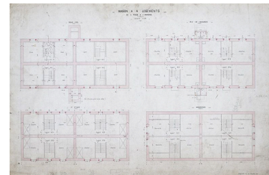
Maison à quatre logements de 4 pièces et une mansarde. Plan du sous-sol, du rez-de-chaussée, du 1er étage et des mansardes. Plan, encre, lavis, échelle 1/50, Lafeschotte, 26 novembre 1919. Phot. Jérôme Mongreville IVR43_20122501212NUC4A
