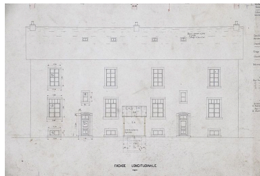
Maison à quatre logements de 4 pièces et une mansarde. Façade longitudinale. Plan, encre, lavis, échelle 1/50, Lafeschotte, 26 novembre 1919. Phot. Jérôme Mongreville IVR43_20122501211NUC4A
